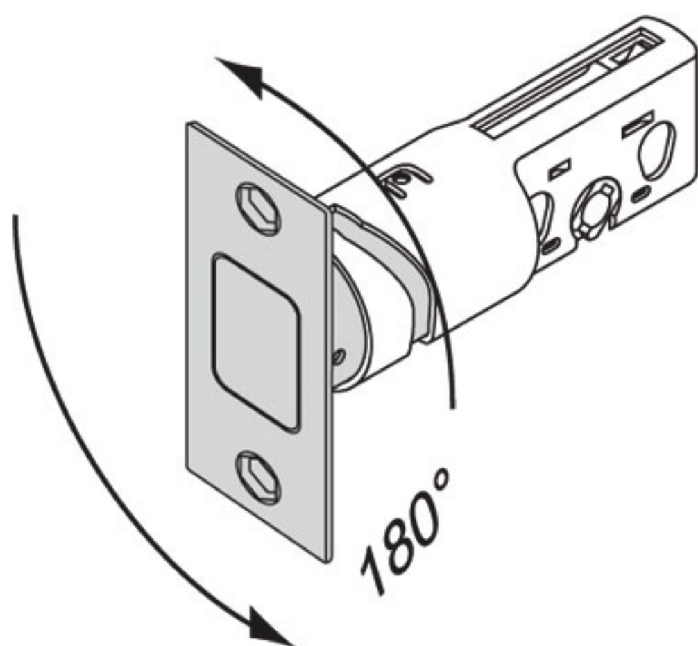
Регулируемая длина ригеля (60-70 мм) для замков SHS-3320/3321
