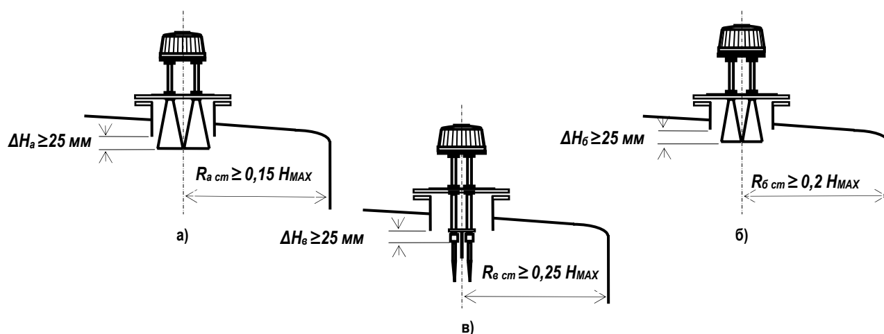
Рисунок 3 - Рекомендуемые варианты монтажа приборов с различными антеннами а) рупорная антенна с диаметром раскрыва 145 мм; б) рупорная антенна с диаметром раскрыва 120 мм; в) стержневая антенна ( H_{MAX} – высота резервуара относительно монтажного фланца прибора, R_{cm} – расстояние от стенки резервуара)
