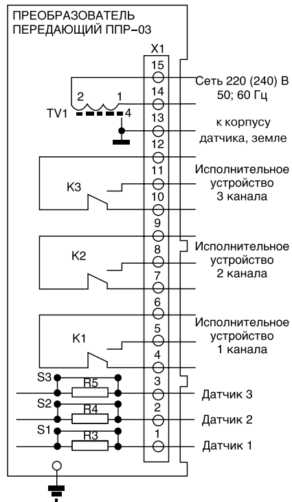
Рис.3 Схема электрическая подключения датчика-реле РОС 301
