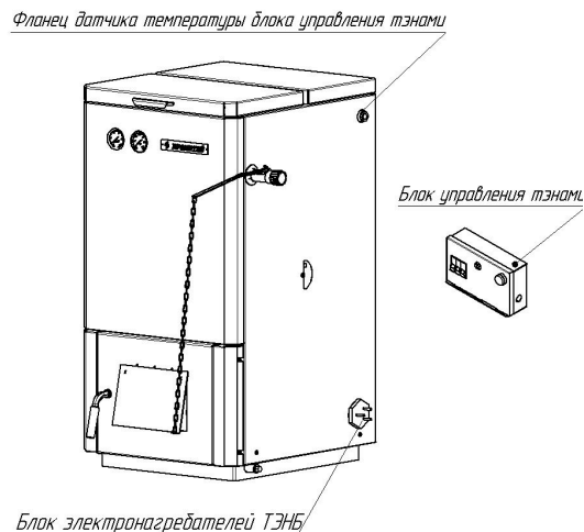
Рис. 7 Подключение блока электронагревателей
