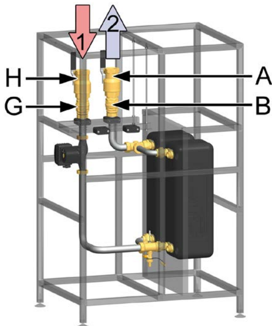
Primärkreis
