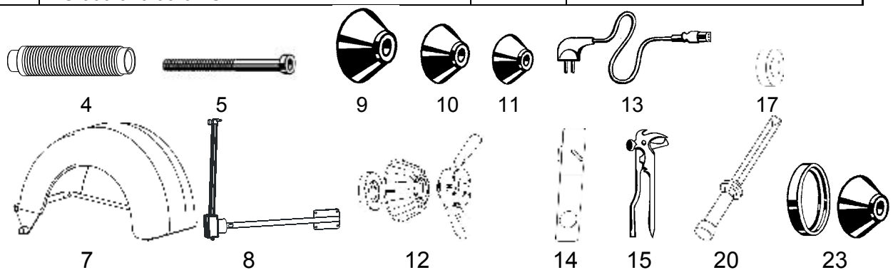
Рисунок 3.1 – Поставляемые принадлежности
