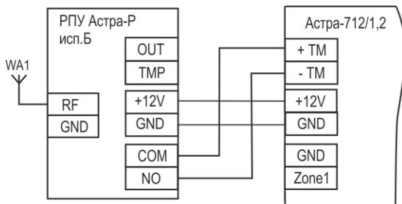
Рисунок А.1- Схема подключения «РПУ Астра-Р» исполнение Б
