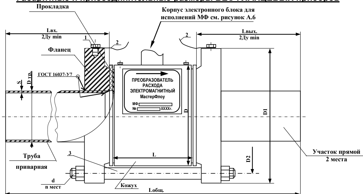
Рисунок А.3 – Поставка бесфланцевых приборов исполнения МФ-2.2Х.Х с комплектом монтажных частей КМЧ МФ №2 с прямыми участками трубопровода, или КМЧ МФ №1 без прямых участков трубопровода
