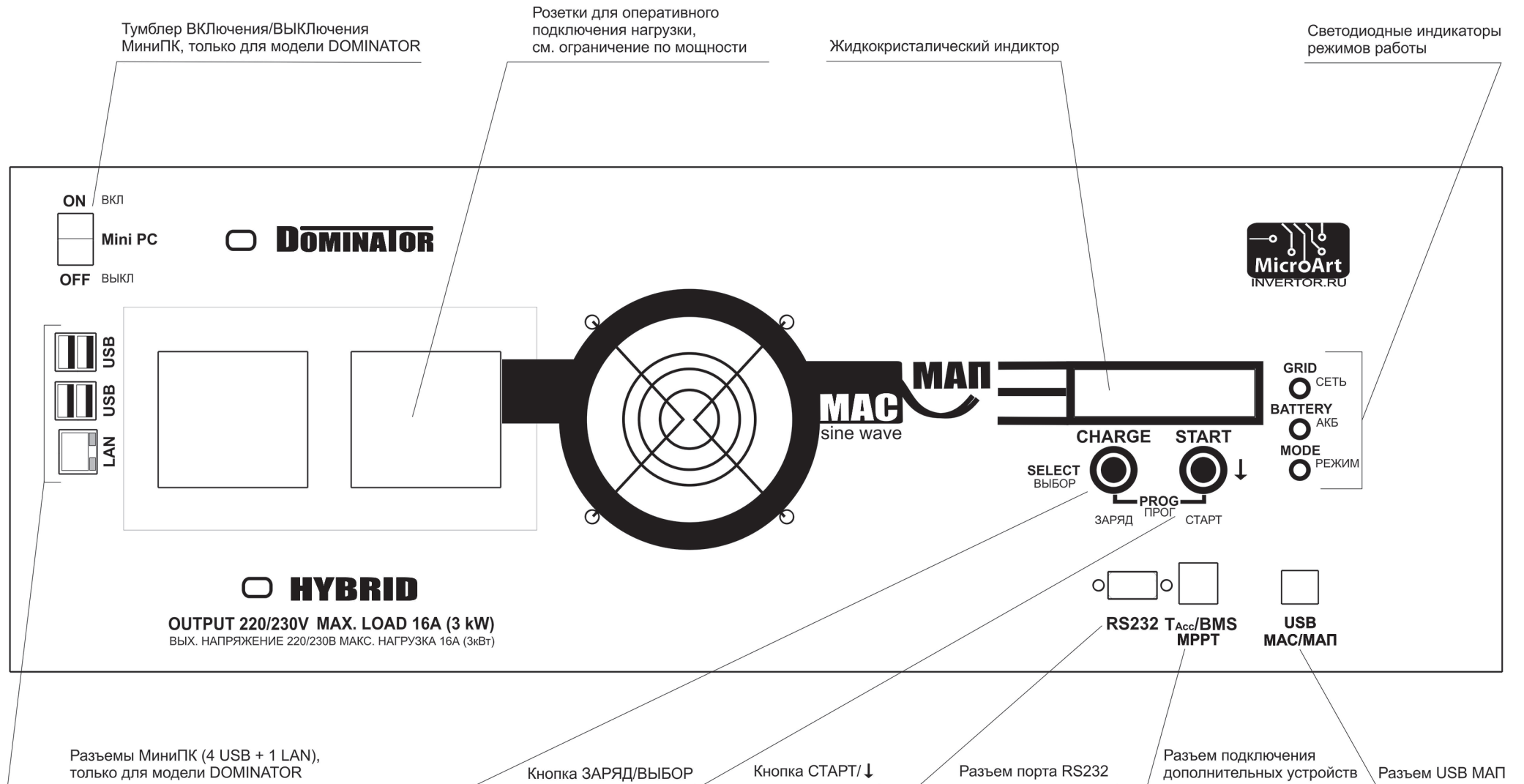
Рисунок 1. Внешний вид инвертора, лицевая сторона
