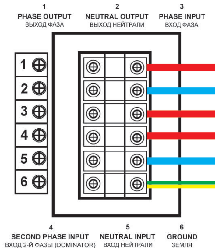
Рисунок 5. Клеммная колодка приборов мощностью от 3 кВт.
