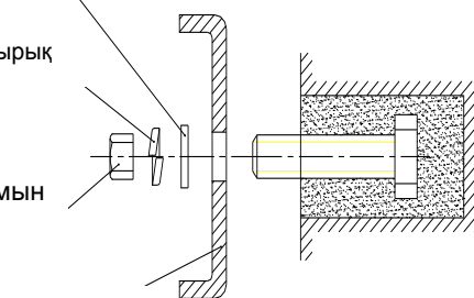
Монтаждау пластинасы
