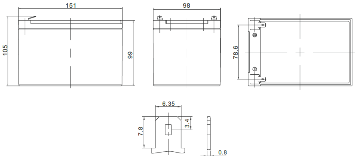
F2 Terminal
