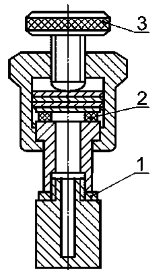
1 — металлическая прокладка; 2 — испытуемый образец; 3 — зажимной винт
