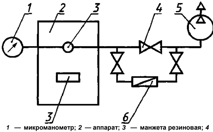
1 — микроманометр; 2 — аппарат; 3 — манжета резиновая; 4 — кран проходной; 5 — вакуум-насос; 6 — расходомер Рисунок 1 — Схема проверки аппарата на герметичность
