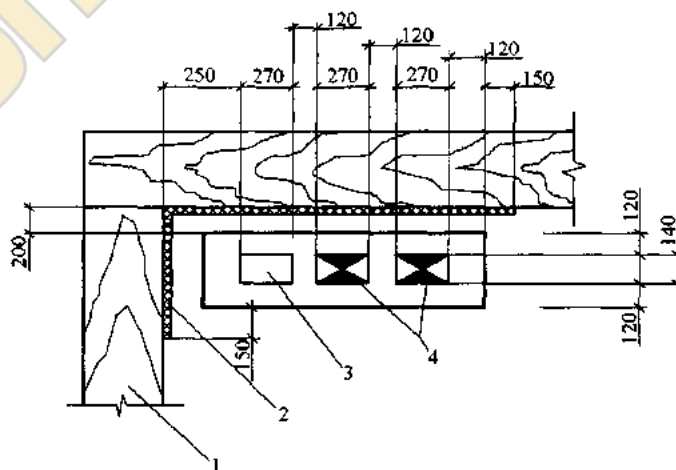
Рис. 6.11. Устройство отступки:
