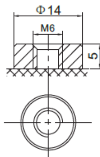
F11 TERMINAL
