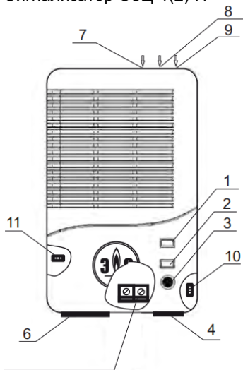
Сигнализатор СЗЦ-1(2)-П
