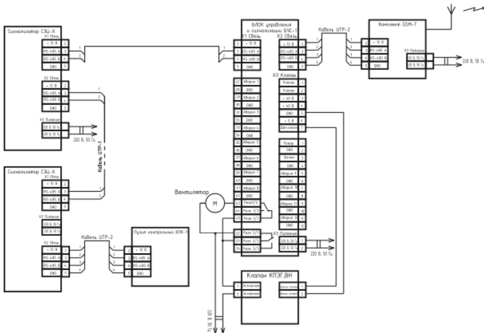
Система контроля «Кристалл-3» с клапаном КПЭГ и дополнительными устройствами (схема электрическая принципиальная)
