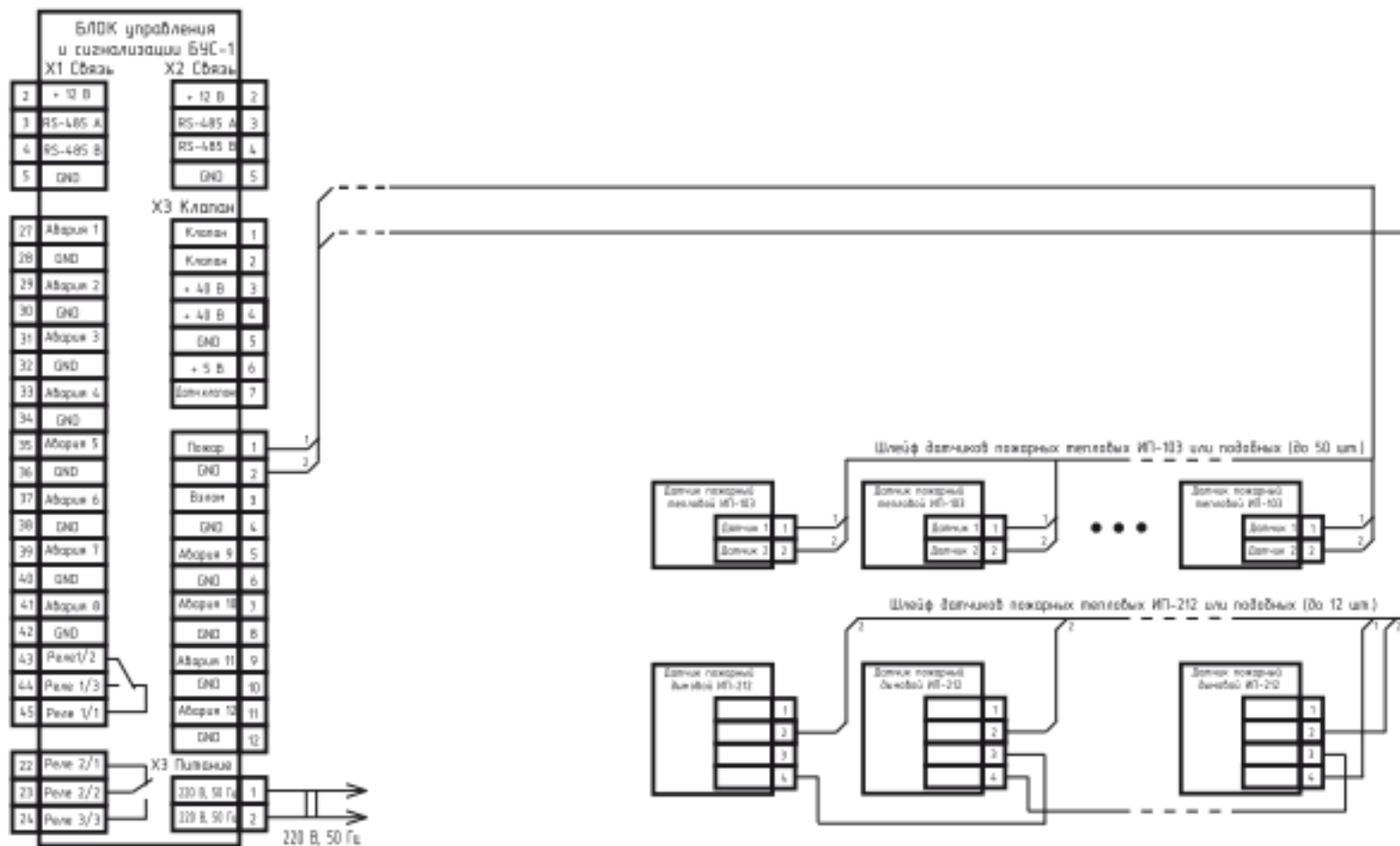
Блок управления и сигнализации БУС-1 с пожарными извещателями (схема электрическая принципиальная)
