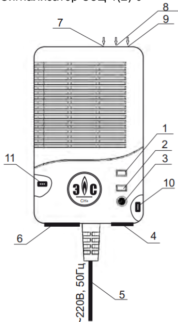
Сигнализатор СЗЦ-1(2)-К.Р.С
