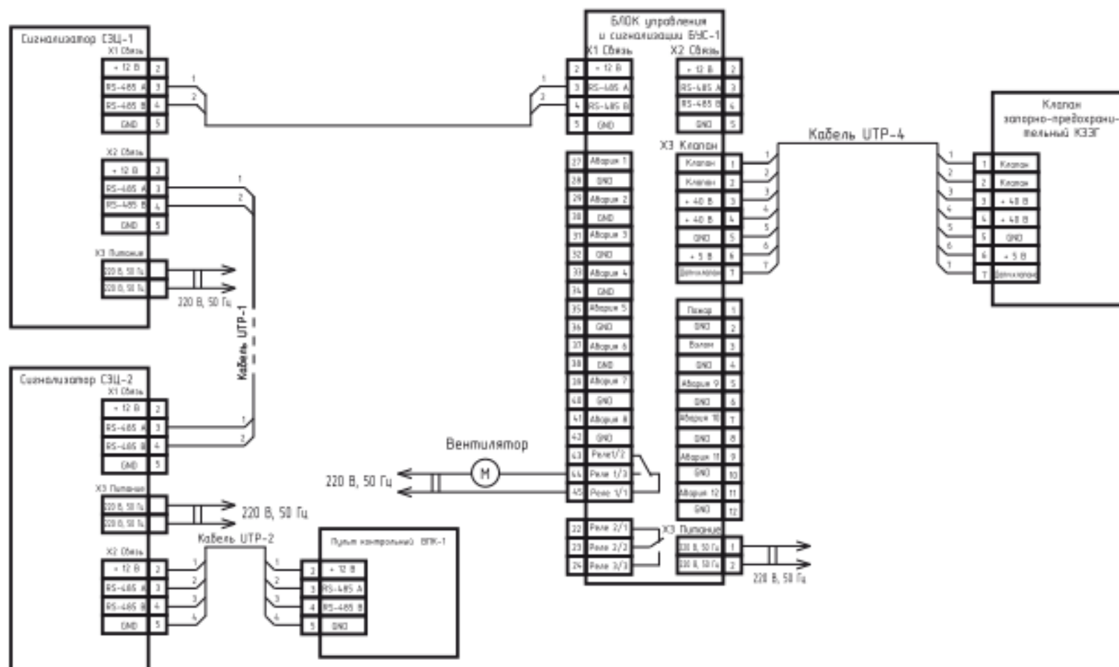
Система контроля загазованности «Кристалл-3». Стандартная комплектация (схема электрическая принципиальная)
