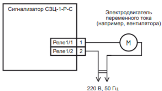
Подключение дополнительных устройств к сигнализаторам СЗЦ-...-Р-С
