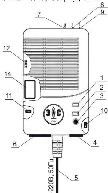
Сигнализатор СЗЦ-1(2)-П
