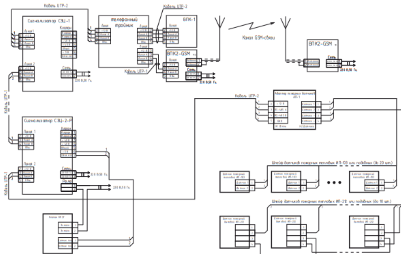
Система «Кристалл-2» с опциями (схема электрическая принципиальная)
