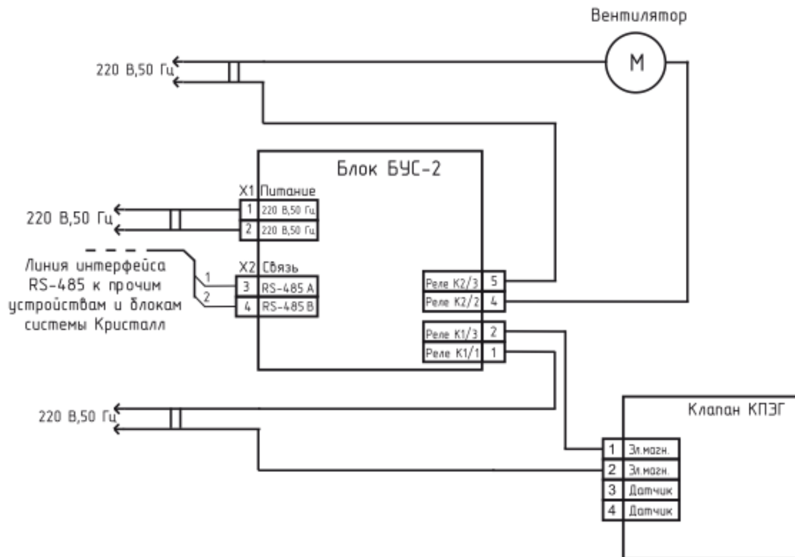
Подключение исполнительных устройств к системе контроля загазованности «Кристалл» с помощью блока БУС-2 (схема электрическая принципиальная)
