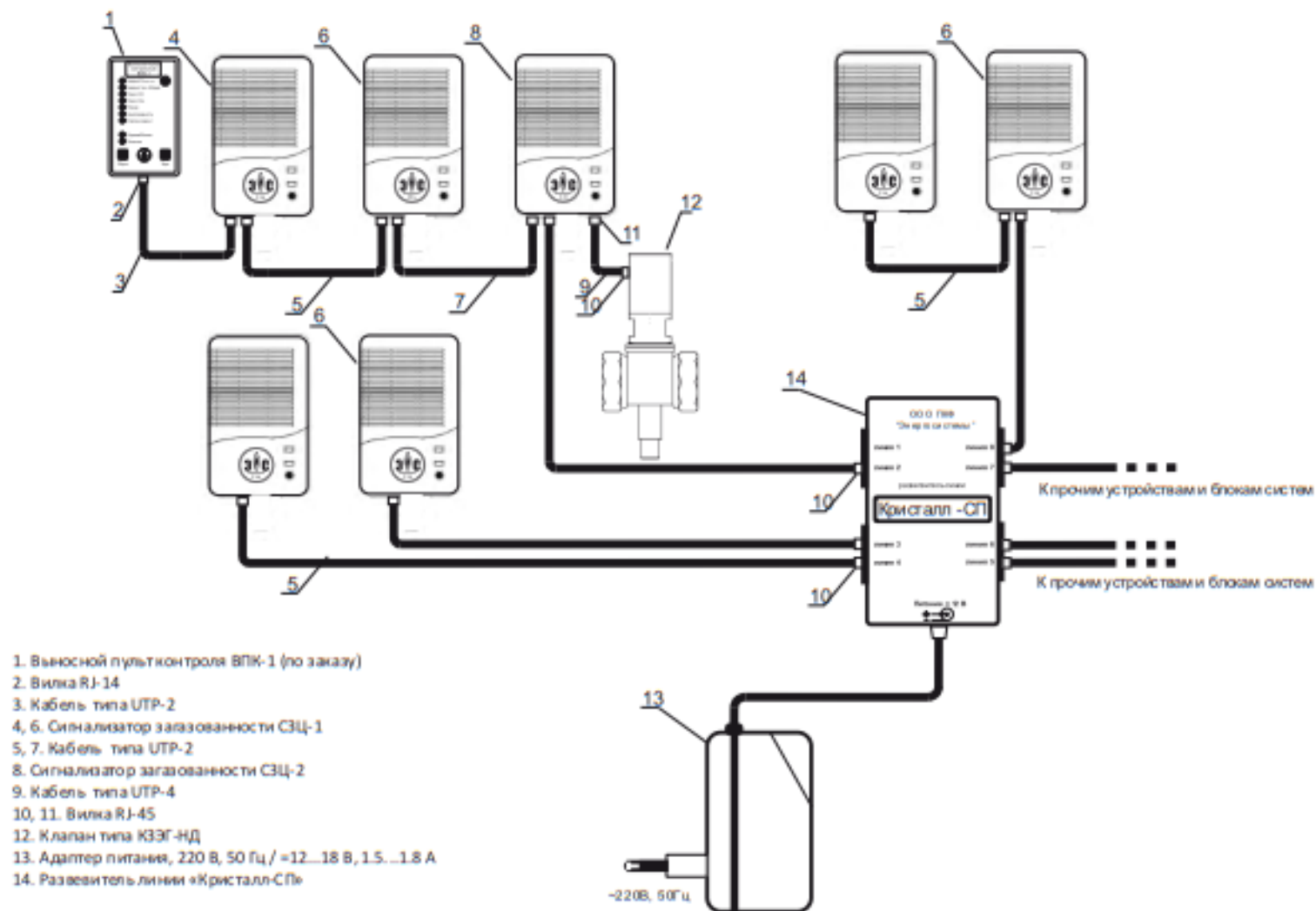
Система контроля загазованности СКЗ «Кристалл» с выносным пультом контроля ВПК-1 (с клапаном КЗЭГ-НД), питанием сигнализаторов постоянным током и переходом от шинной структуры связей к радиальной
