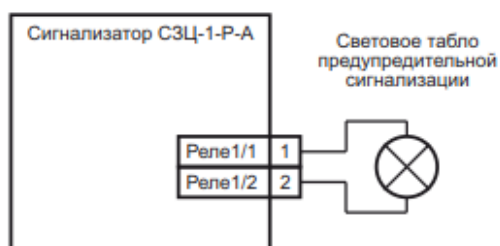
Подключение светового табло к сигнализатору СЗЦ-...-Р-А
