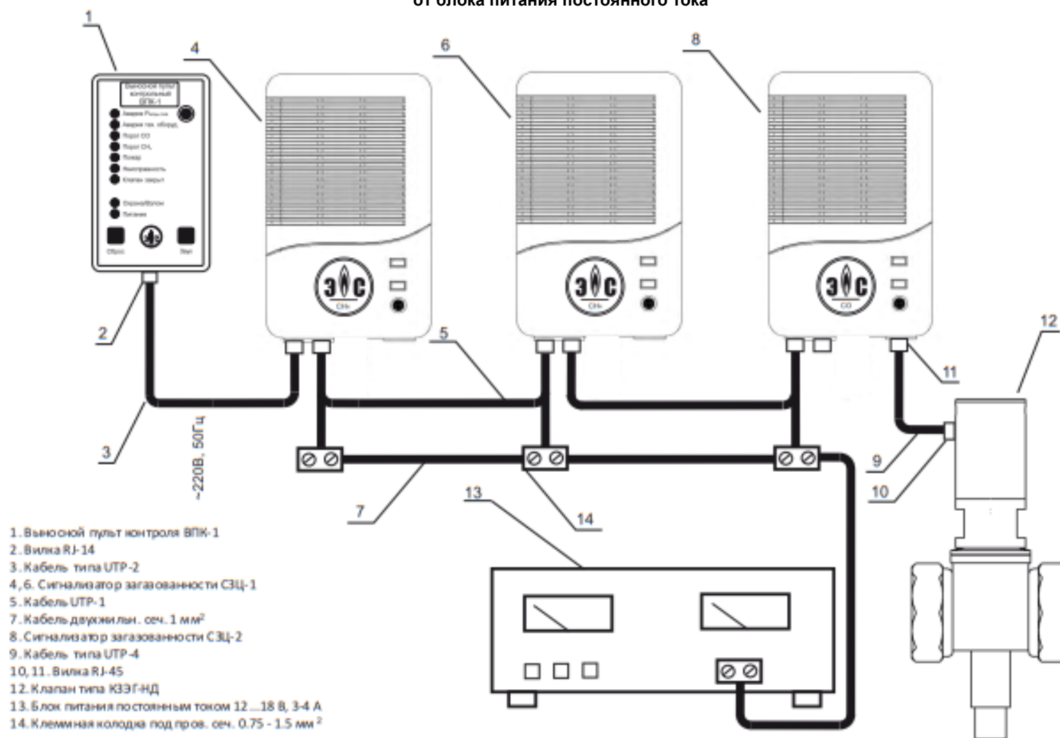
Система контроля загазованности СКЗ «Кристалл-2» с выносным пультом контроля ВПК-1 (с клапаном КЗЭГ-НД) и питанием постоянным током от блока питания постоянного тока
