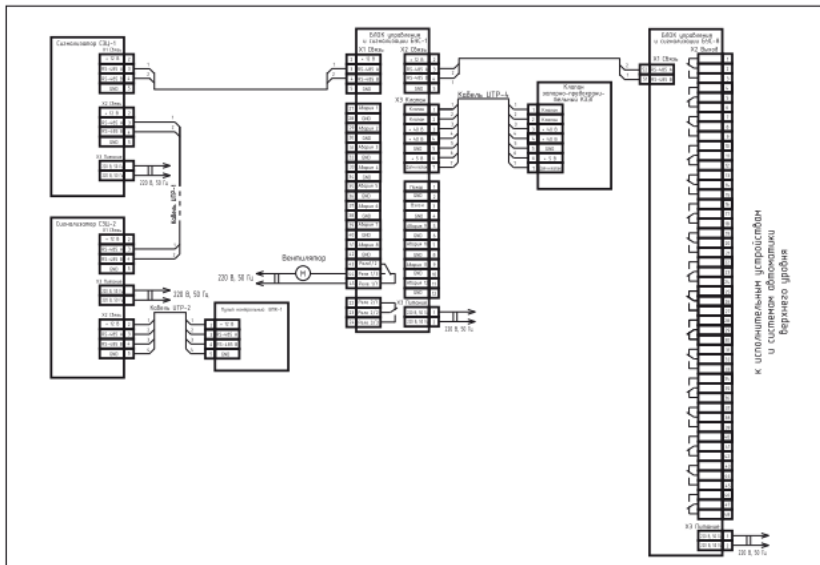
Система контроля загазованности «Кристалл-3» с блоком управления БУС-8 (схема электрическая принципиальная)
