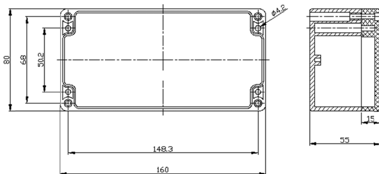
Рис. Д2 Габаритные и присоединительные размеры котроллера ВК-2.1
