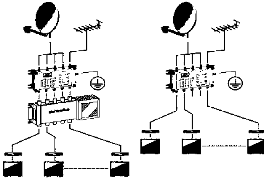
Рисунок 12- Антенна с блоком схемы защиты
