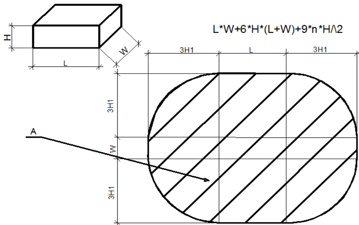
А.1-суреті – Тікбұрышты ғимарат
