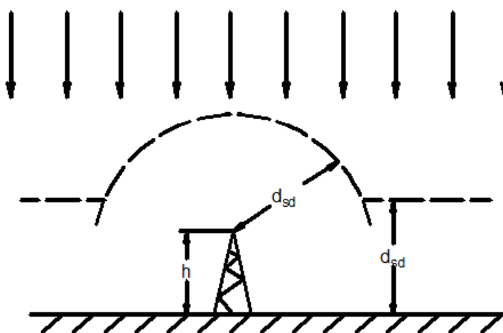
4-сурет – электр геометриялық әдіс бойынша объектіге түскен найзағай санын бағалау
