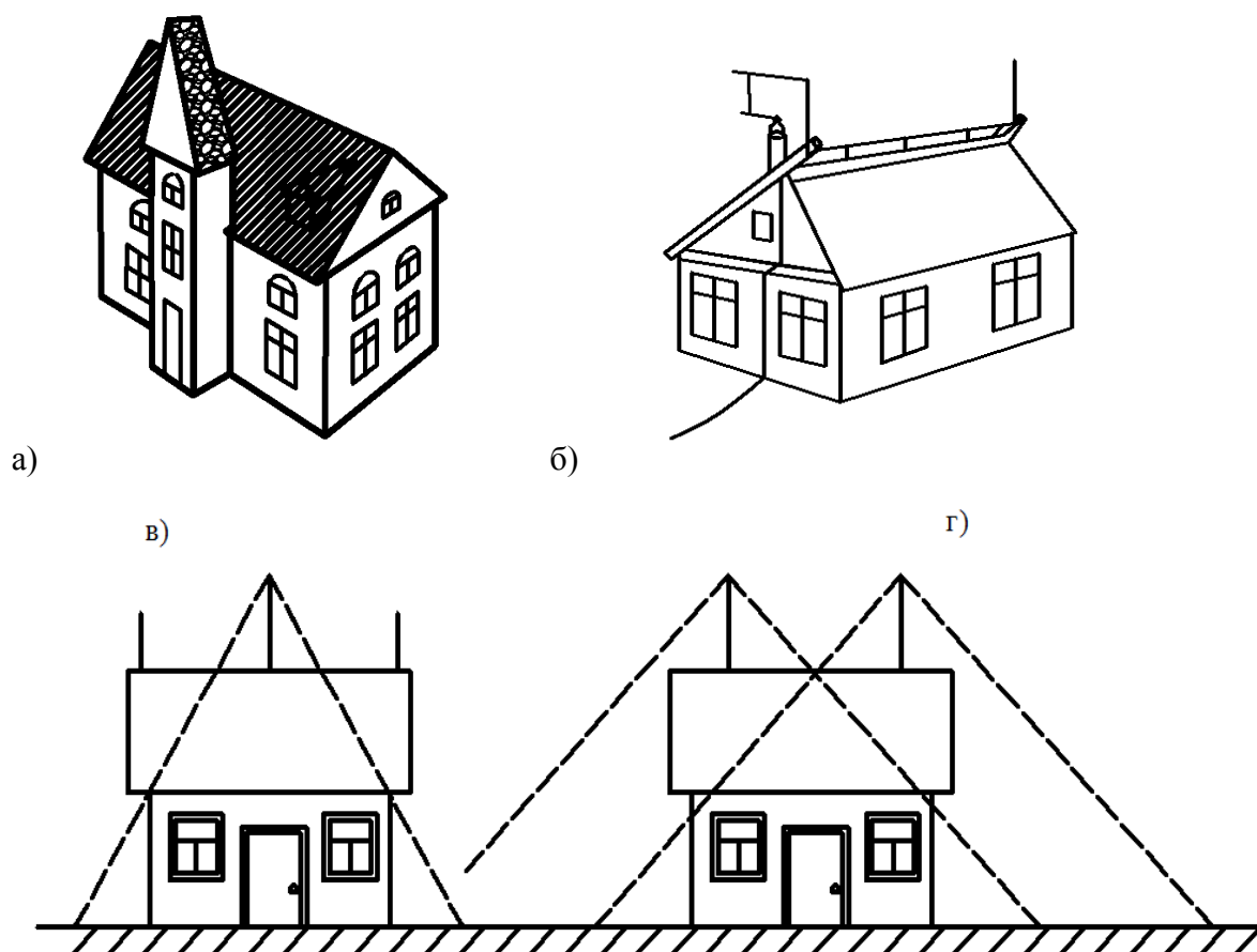
6-сурет – Жобадағы (б) үй көлденеңі мен күн күркіреуді бұрғыштың (а) қорғаныс аймағы
