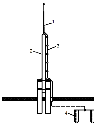
8-сурет – Өзекшелі дара тұрған найзағай бұрғыш
