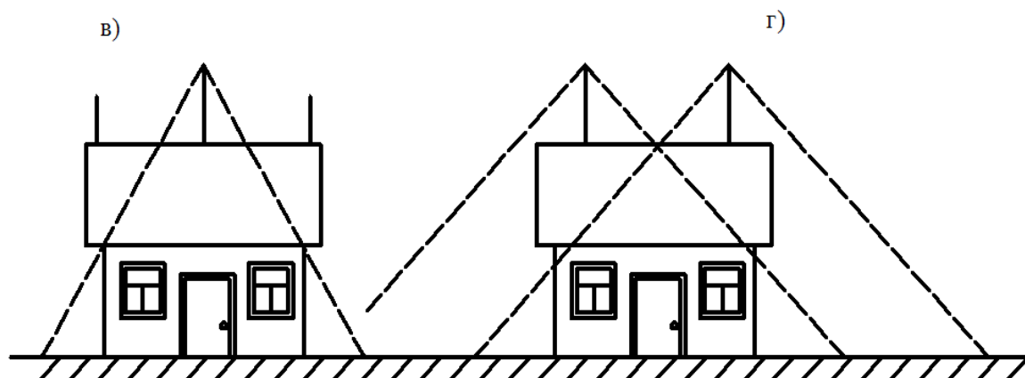
а — молниеотвод на самой высокой части дома; б — горизонтальный (тросовый) молниеприемник; в — дополнительные молниеприемники на фронтонах; г — два разнесенных молниеприемника
