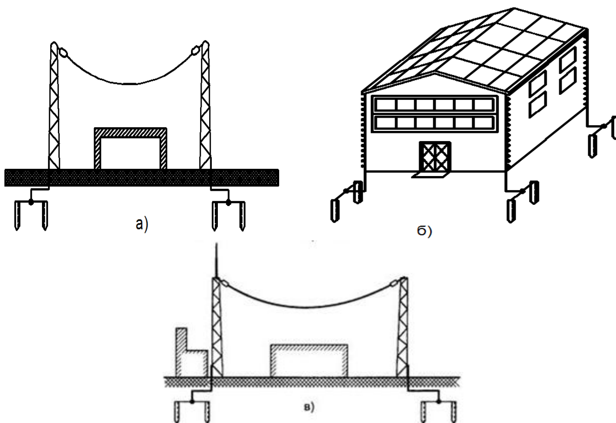
9-сурет – Арқанды және тор қабықты найзағай бұрғыштар
