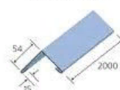
Конек узкий
