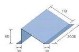
Снегозадержатель
