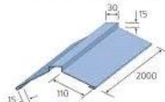
Конек прямоугольный
