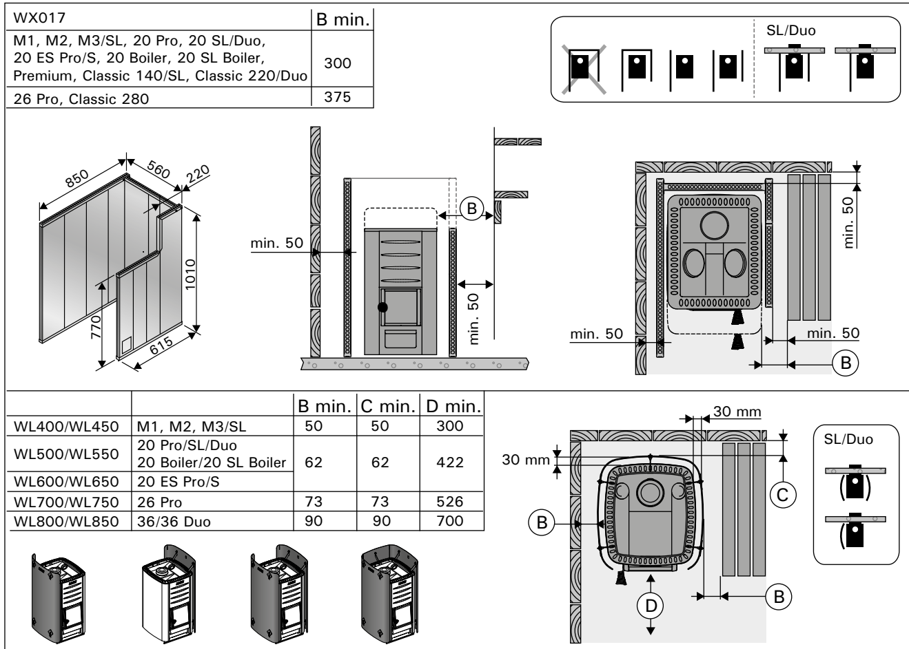
Рисунок 8. Безопасные расстояния с защитными ограждениями (все размеры приведены в миллиметрах) Joonis 8. Ohutuskaugus koos kaitseseinaga (kõik mõõtmised millimeetrites)
