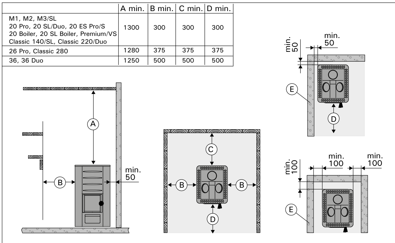
Рисунок 7. Безопасные расстояния (все размеры приведены в миллиметрах) Joonis 7. Ohutuskaugused (kõik mõõtmised millimeetrites)
