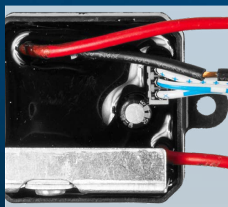
Электронный блок управления с полной заливкой для защиты от пыли
