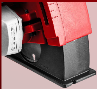
Автоматически закрывающийся кожух защищает оператора и уменьшает распространение пыли
