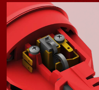
Специальная конструкция щеткодержателя для защиты коллектора при полном износе щеток
