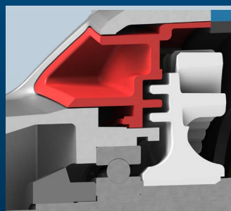
Лабиринтные уплотнения подшипников исключают попадание пыли и выход из строя
