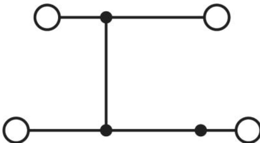
Электрическая схема
