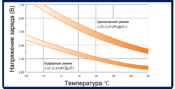
Зависимость между напряжением заряда и температурой
