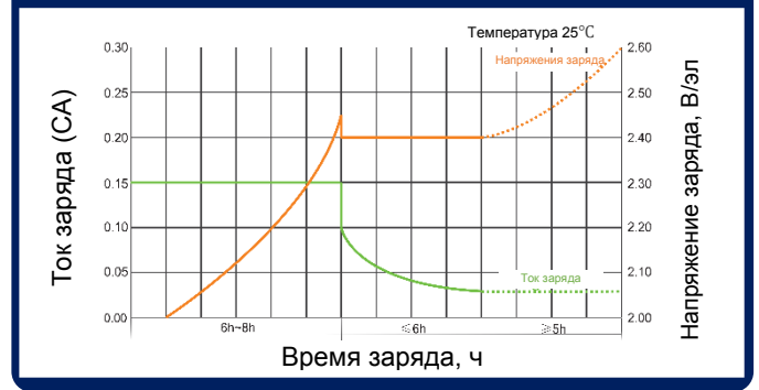
График заряда (IUI)
