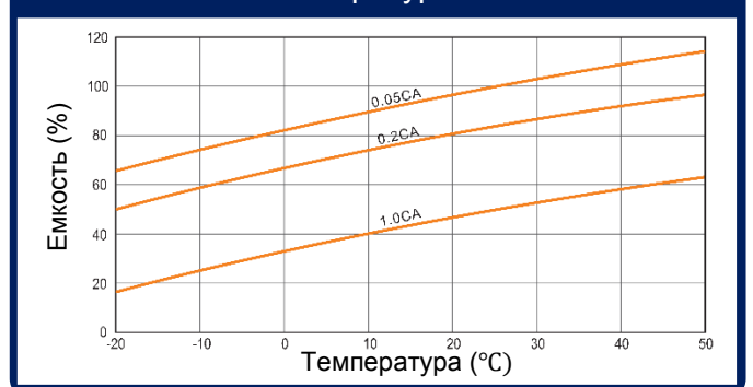
Влияние температуры на емкость
