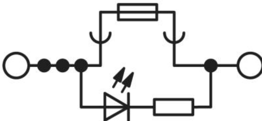
Электрическая схема
