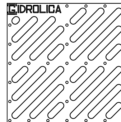
Решетка чугуная щелевая кл. С250
