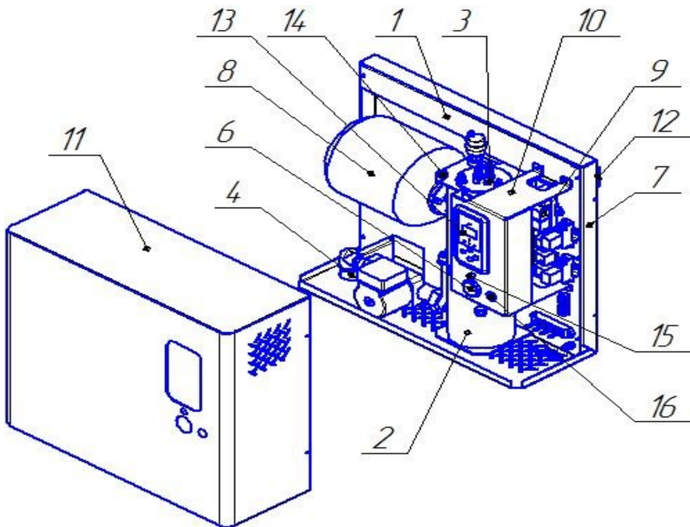
Рис.1 Конструкция электроводонагревателя
