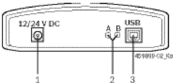
Fig. 2: Соединительный выход 1 Соединение переходного кабеля с батарей или прикуривателем 2 LED A и LED B (См. раздел 3.5.3) 3 USB-соединение
