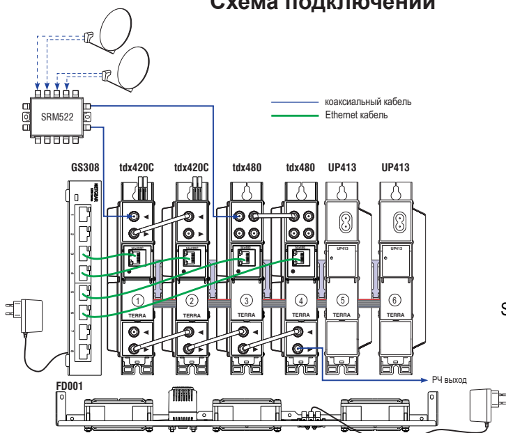
Схема подключений
