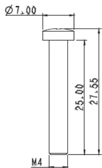
Винт фиксации металлической платы В
