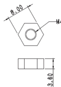
Гайка фиксации металлической платы В
