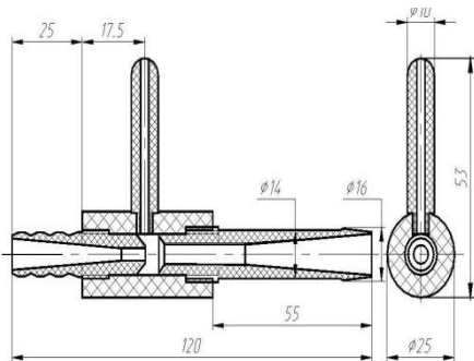
Рис. 26 НВФ-1
