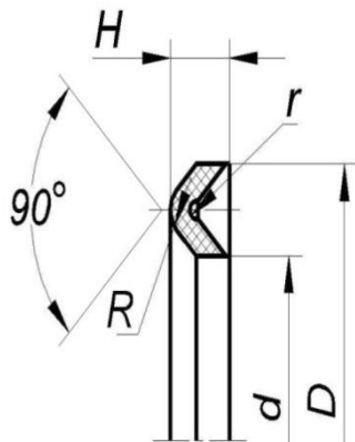
Рис. 18 Манжета
