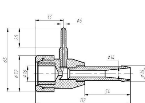
Рис. 27 НВФ-2
