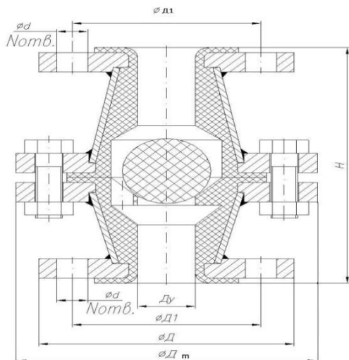
Рис. 24 Клапан обратный шаровый в броне
