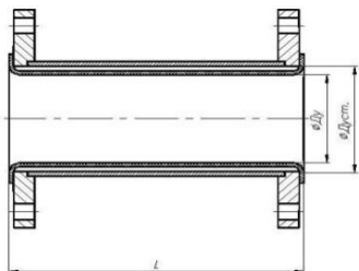
Рис. 1 Труба, футерованная фторопластом-4
