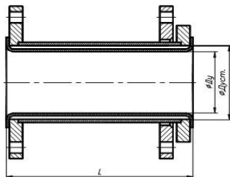
Рис. 2 Трубы с одним и двумя накидными фланцами
