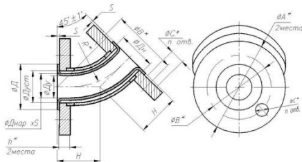
Рис. 9б Отводы с углом 45°
