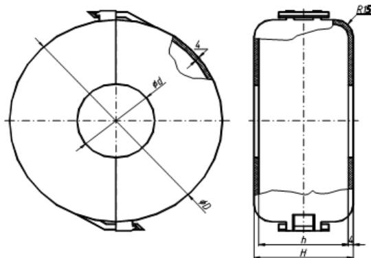
Рис. 33 Кожух защитный
