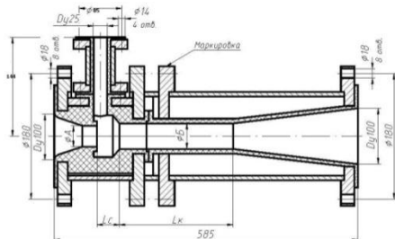
Рис. 21 НСФБ
