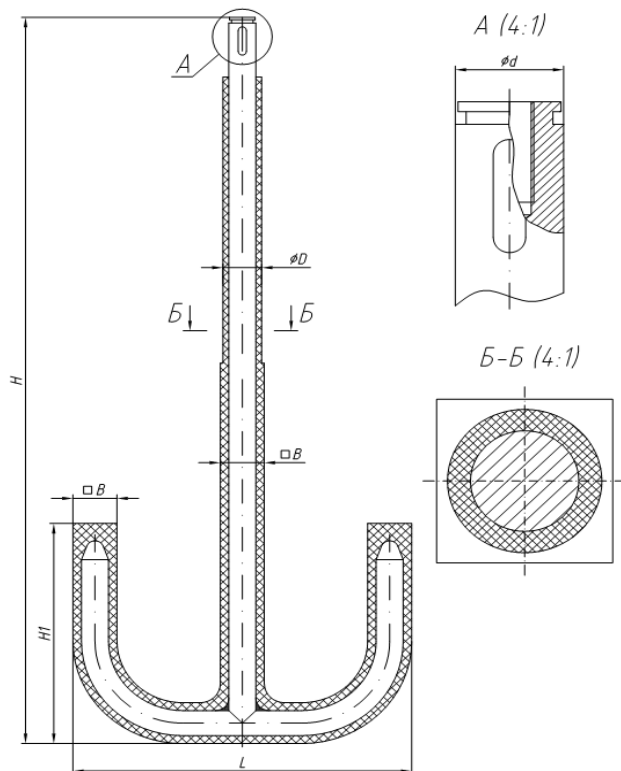
Рис. 34 Мешалка стальная, футерованная фторопластом-4
