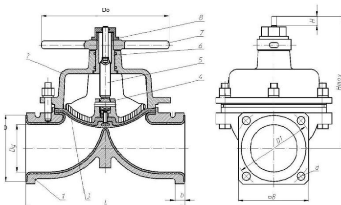
Рис. 15 клапан
