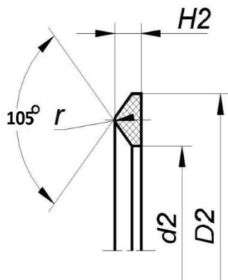
Рис. 19 Кольцо опорное
