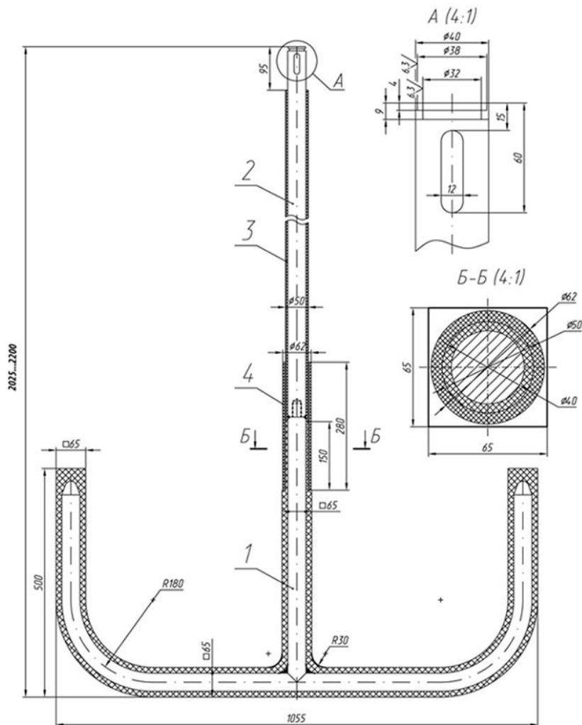
Рис. 36 Мешалка стальная, футерованная фторопластом-4
