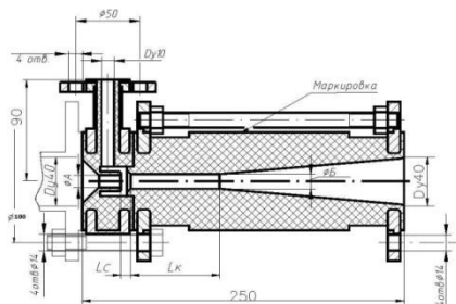
Рис. 22 НСФ2
