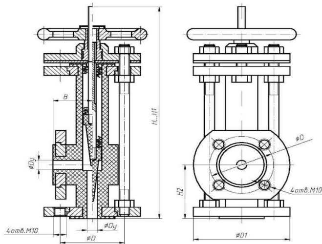
Рис. 25 Вентиль регулирующий сильфонный
