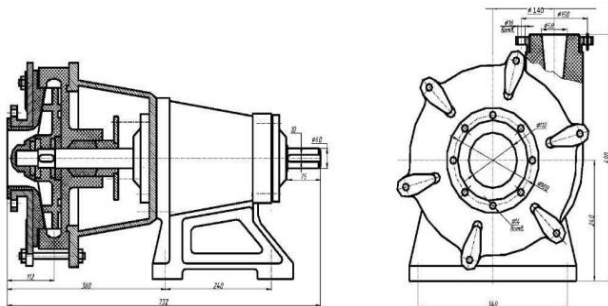
Рис. 28 Насос центробежный марки Х45/23/4-П
