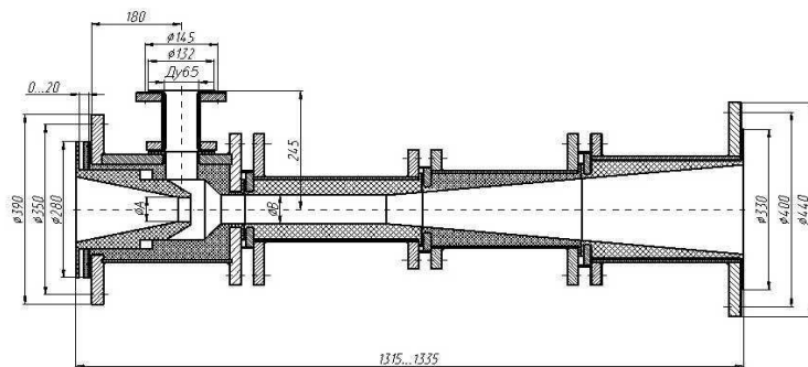
Рис. 23 НСФБЕ
