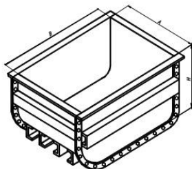
Рис. 29 Ванна, футерованная листами из Ф-4
