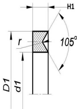
Рис. 17 Кольцо нажимное
