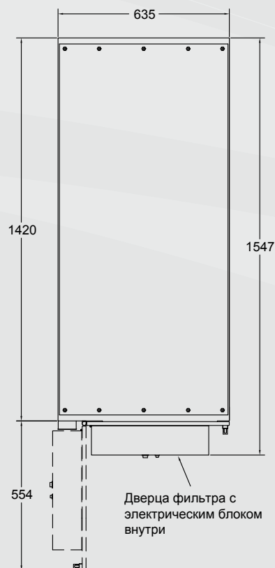
Вид сзади
