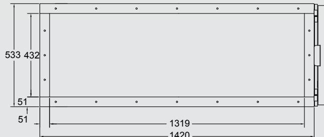
Вид сзади
