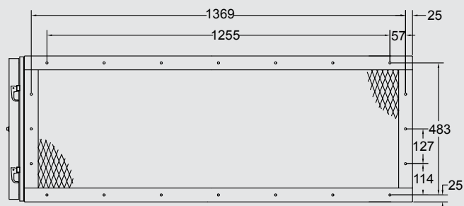
Вид спереди
