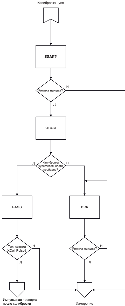
Рис. 12 Калибровка чувствительности
