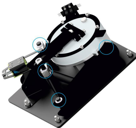
Рисунок 12.5.1 – Места смазки подвижных частей
