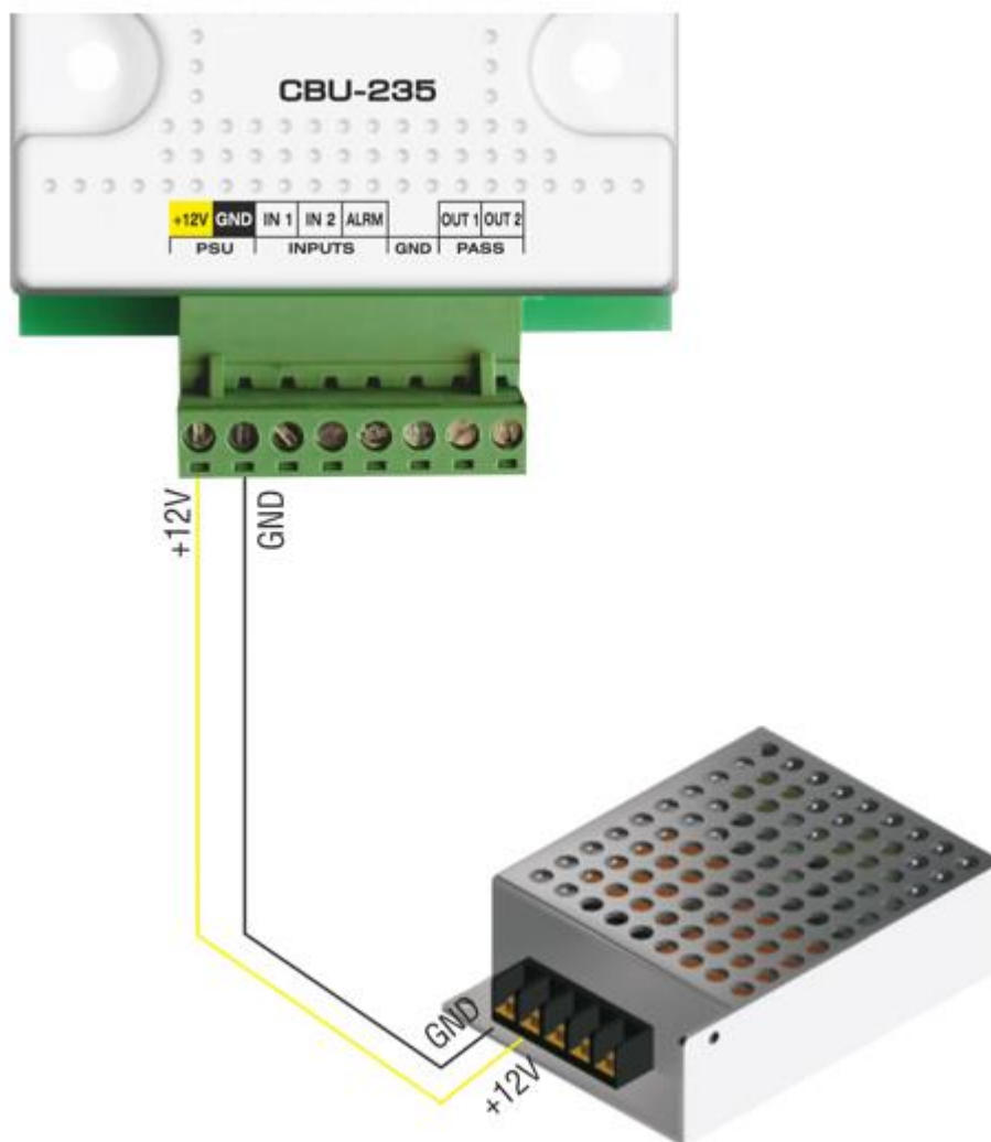
Рисунок 8.4.1 - Подключение питания к турникету
