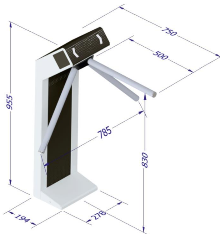
Рисунок 5.1 – Габаритные размеры турникета с планками ЛКД ТТ-12-10.
