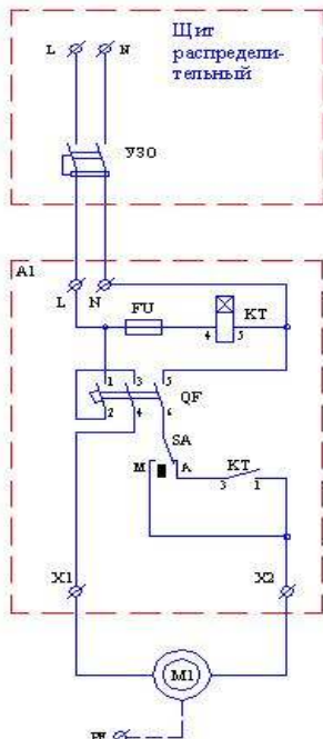
Эл.схема 1
