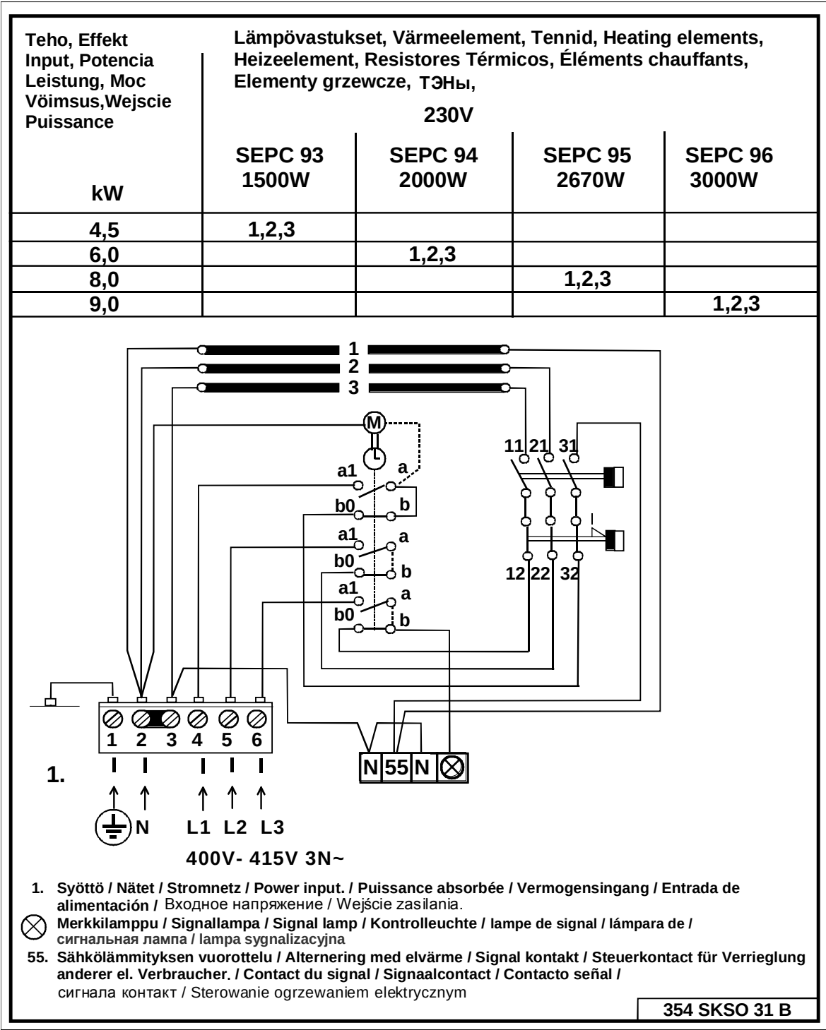
Abbildung 5 Stromlaufplan
