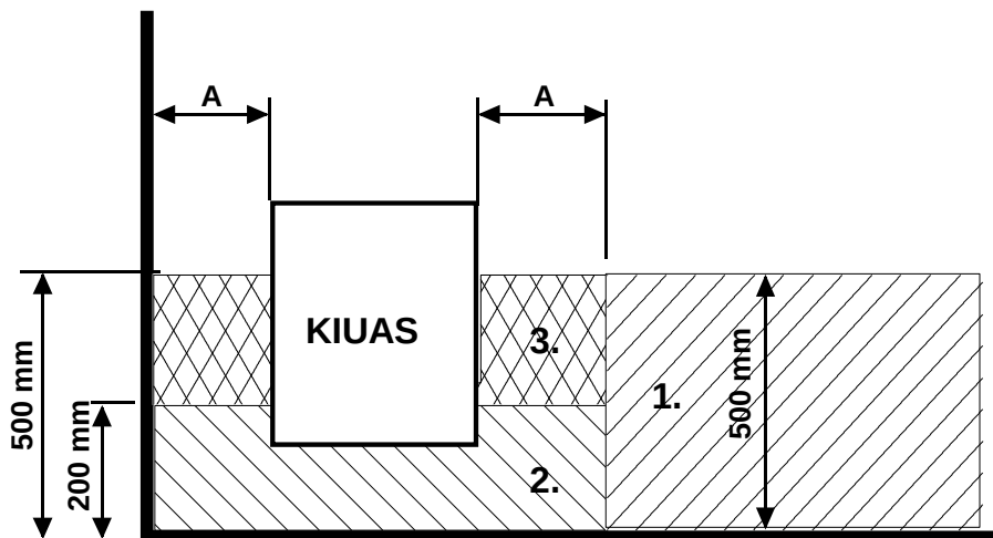
Kuva 4 Kytkentärasian sijoituspaikka
