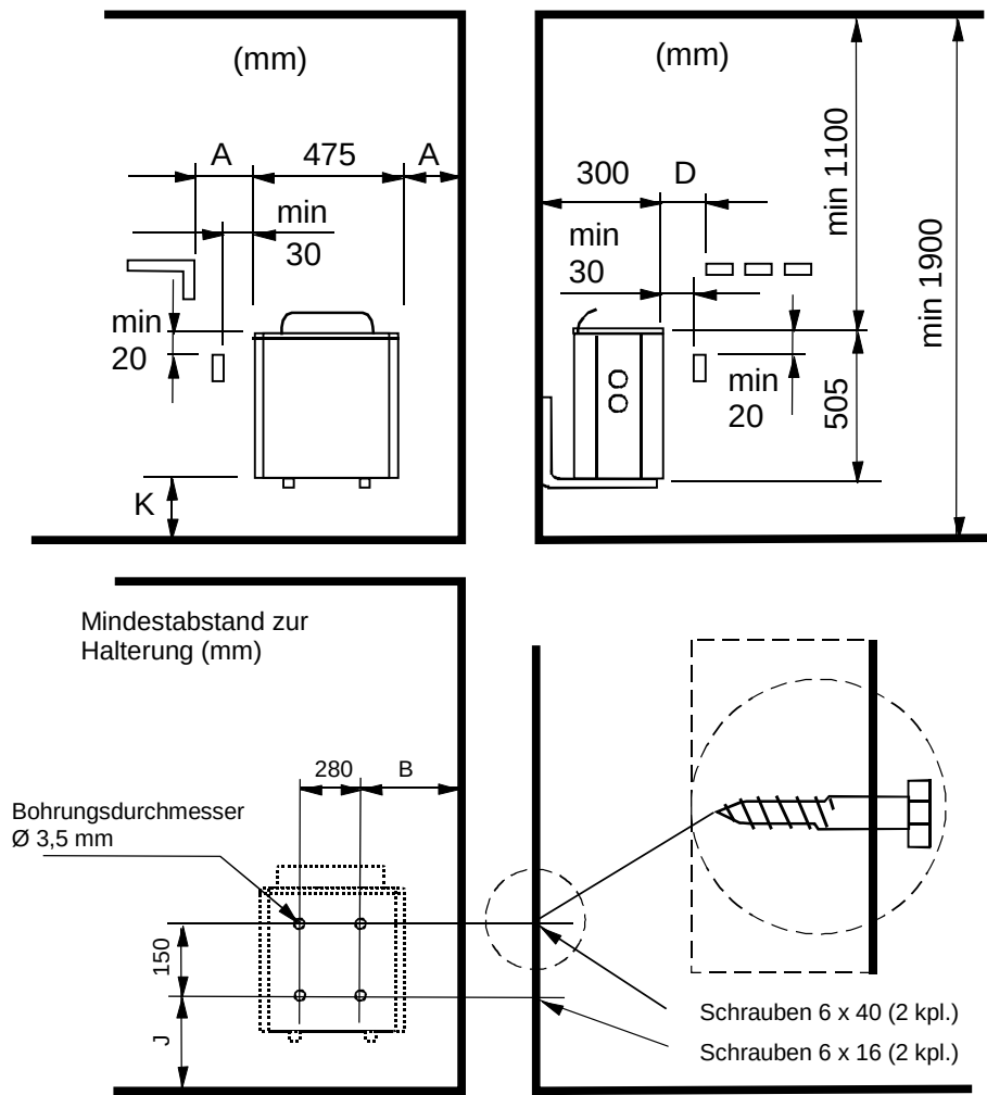
Abbildung 3 Sicherheitsabstände
