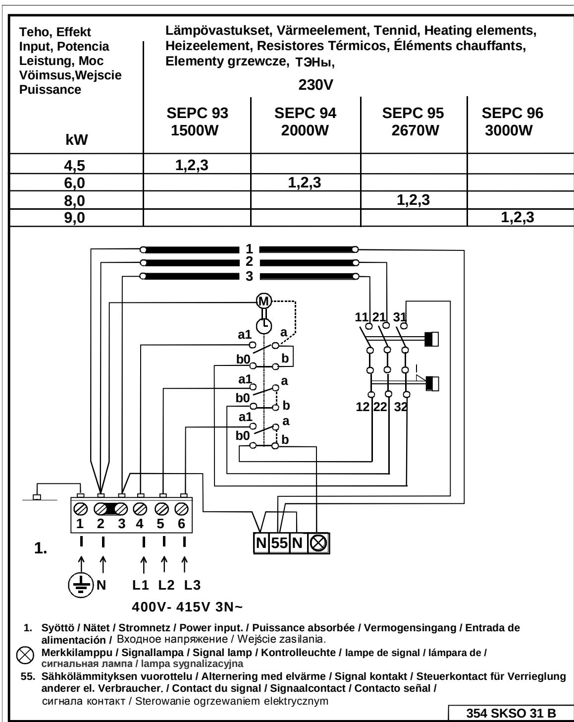
Kuva 5 KytKentäkaava
