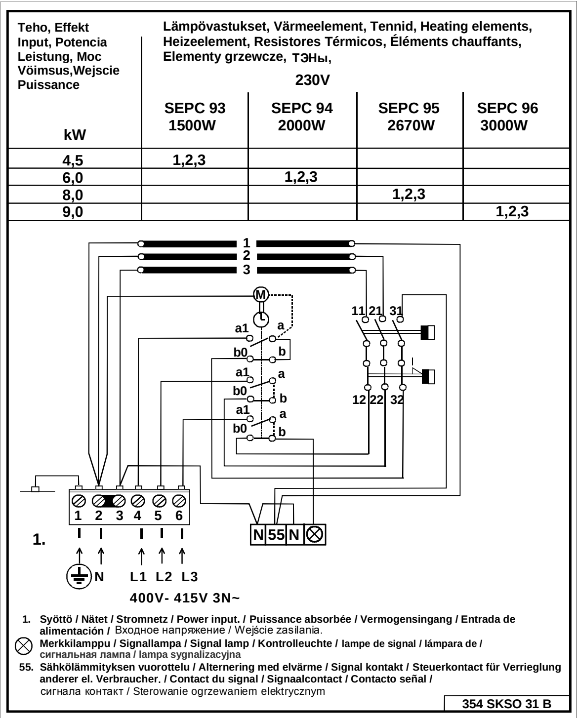
Bild 5 Kopplingsschema
