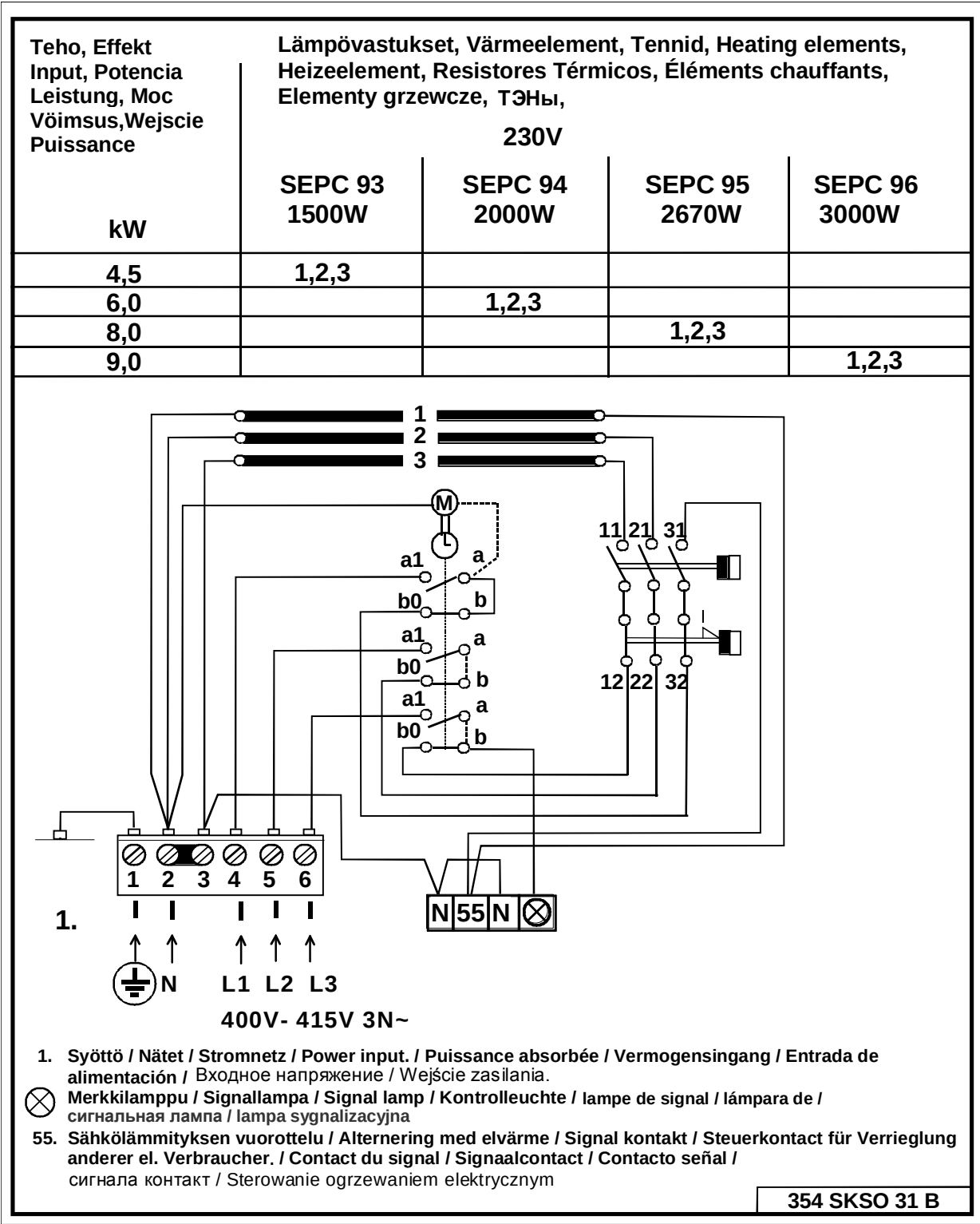
Рисунок 5 Монтажная схема для электрокаменки
