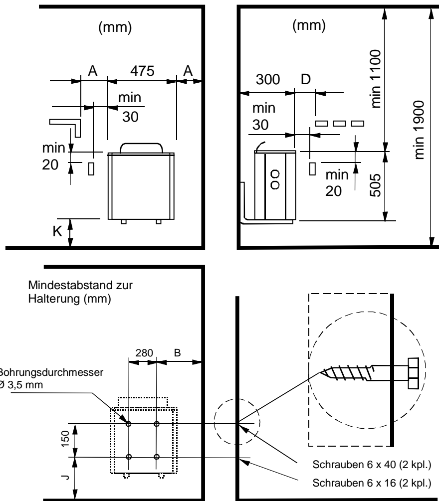
Abbildung 3 Sicherheitsabstände
