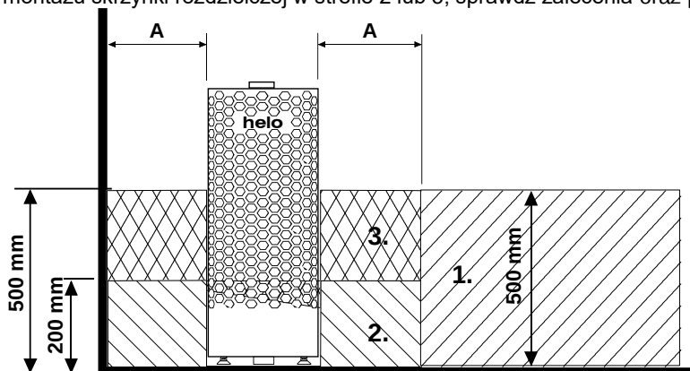
Rysunek 3 Lokalizacja skrzynki rozdzielczej
