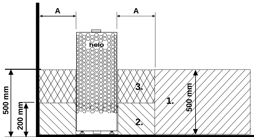
Kuva 3 Kytkentärasian sijoituspaikka
