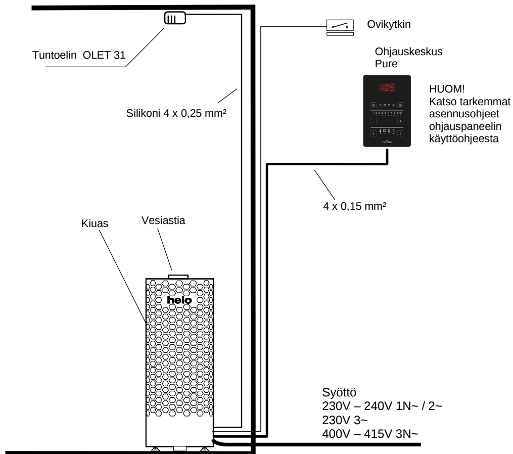
Kuva 9 Periaatekuva kytkennästä
