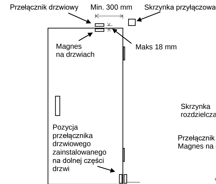
Rysunek 5 Instalacja przełącznika drzwiowego
