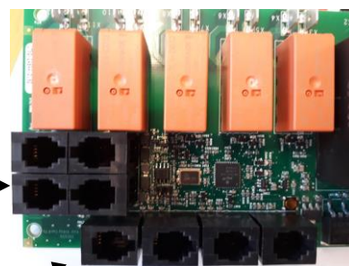
Abbildung 4 . Reihenfolge der RJ 10-Anschlüsse. Sensor, Türschalter, Fernbedienung, zusätzlicher NTC
