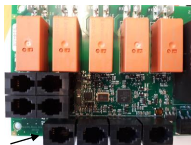
Kuva 4 . RJ 10 liittimien järjestys. Tuntoelin, Ovikytin, Kauko-ohjaus, Lisä NTC
