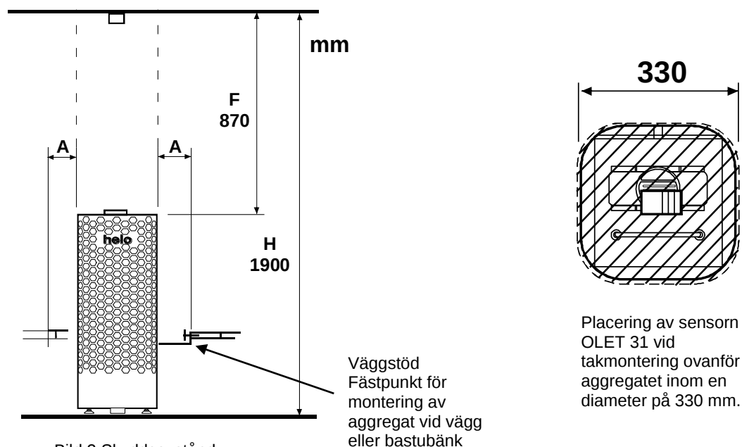
Bild 2 Skyddsavstånd
