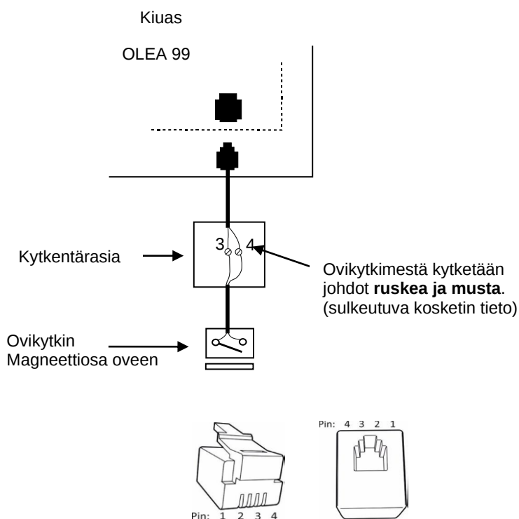
Kuva 6. RJ 10 liittimen Pin -järjestys
