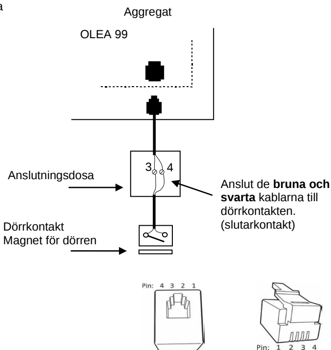
Bild 6 Stift-order av RJ 10
