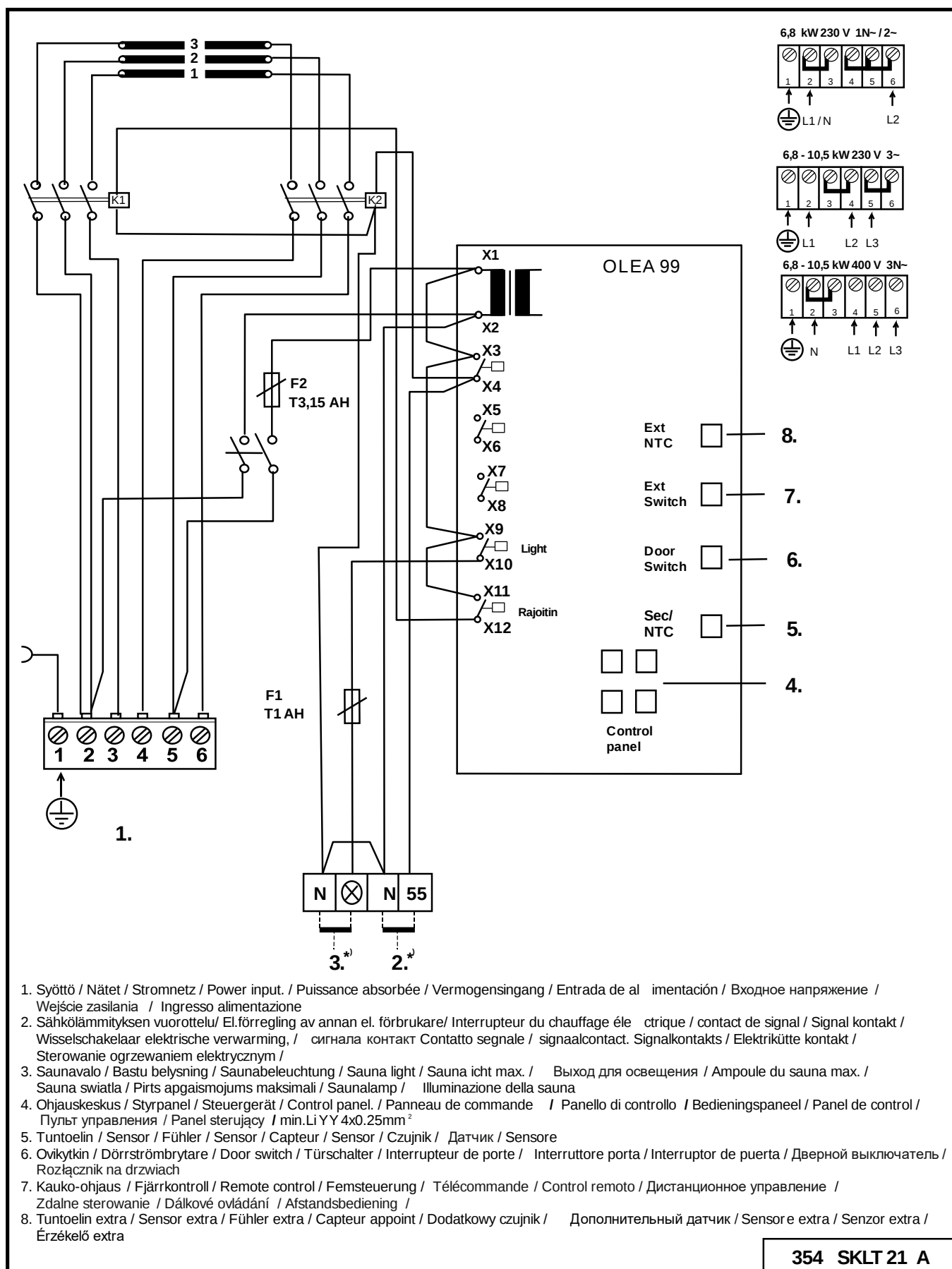
Bild 7 Kopplingsschema
