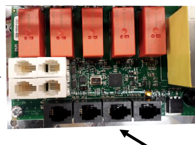
Bild 5 . Ordning på RJ10 -kontakter. Givare, dörrbrytare, fjärrkontroll, extra NTC
