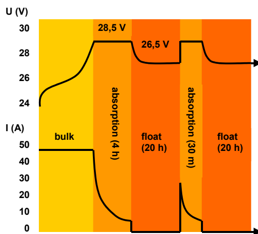
Кривая заряда
