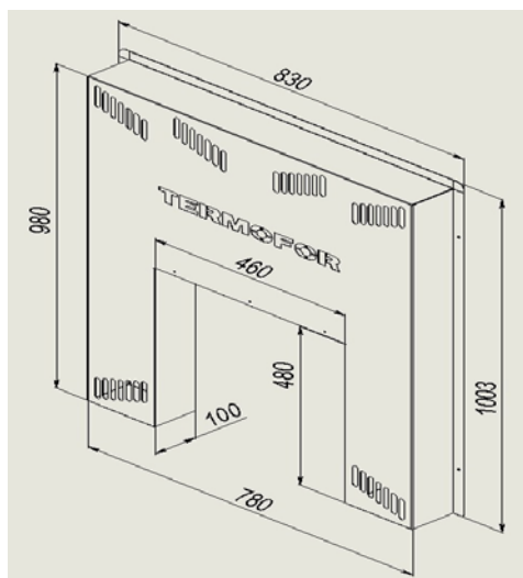
Рисунок 1. Габаритные размеры экрана фронтального Плазма.
