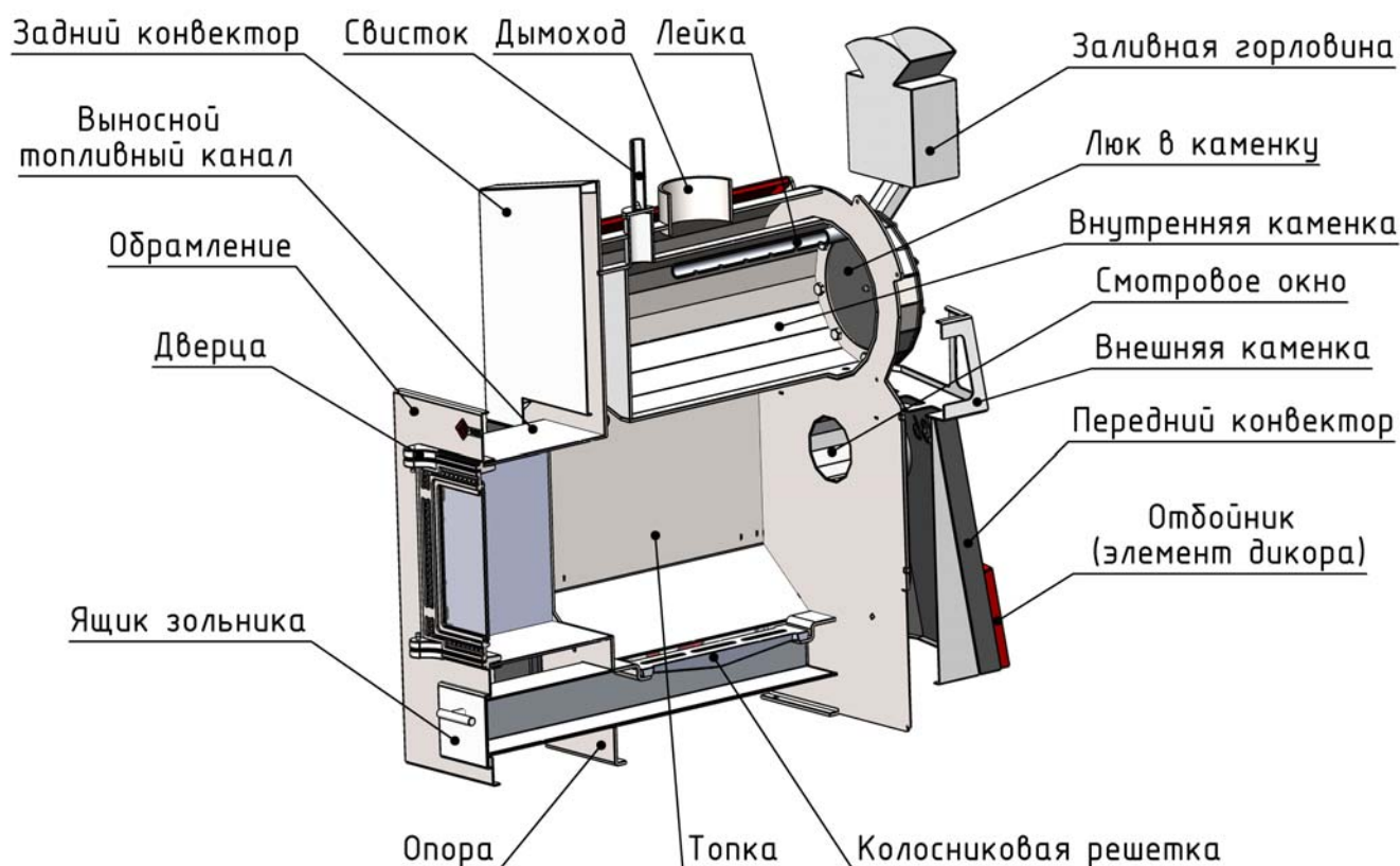
Рис.1- Общий вид в разрезе печи Паровоз
