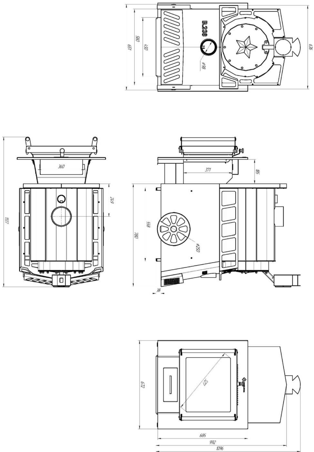
Габаритные размеры печи «Паровоз 18-26 Плазма»
