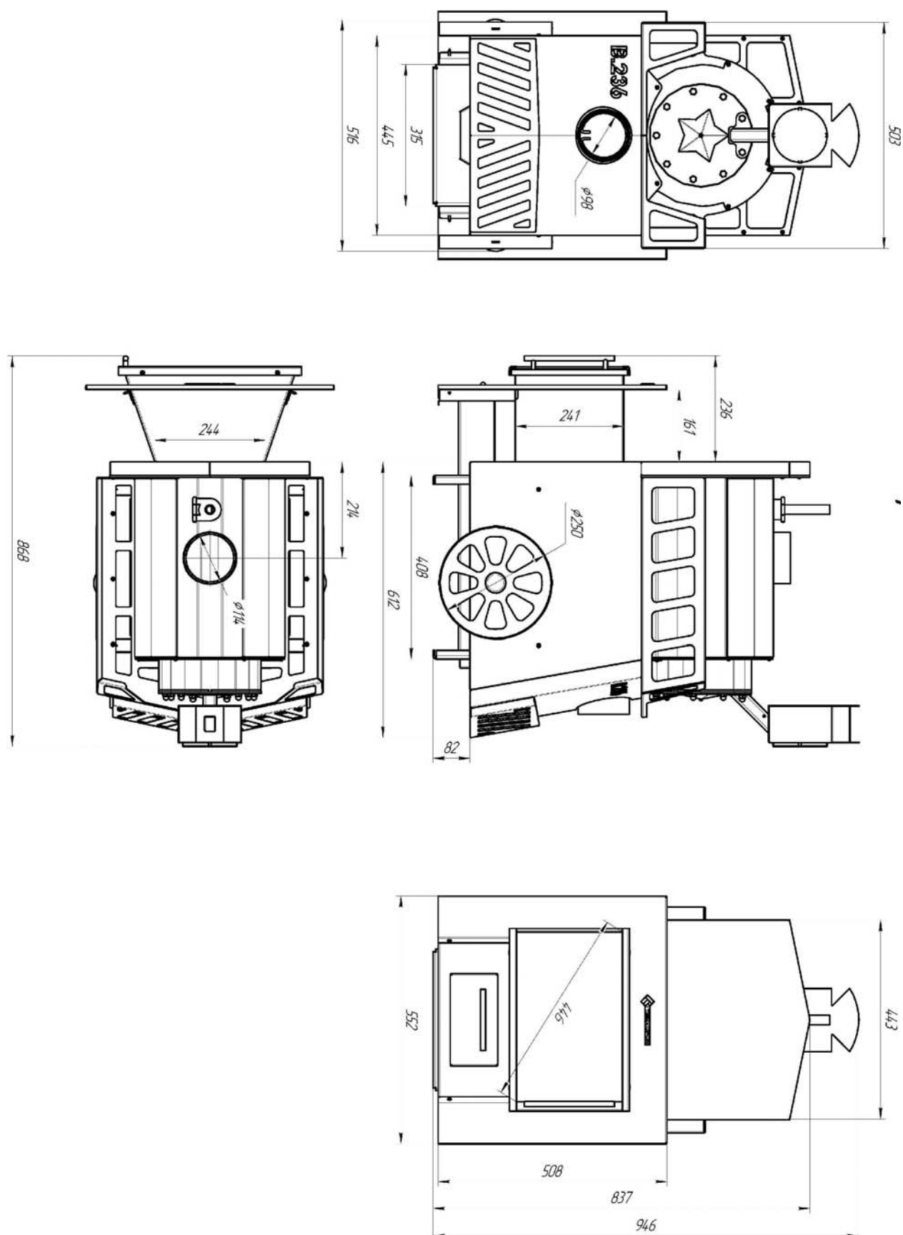
Габаритные размеры печи «Паровоз 9-14 Плазма»
