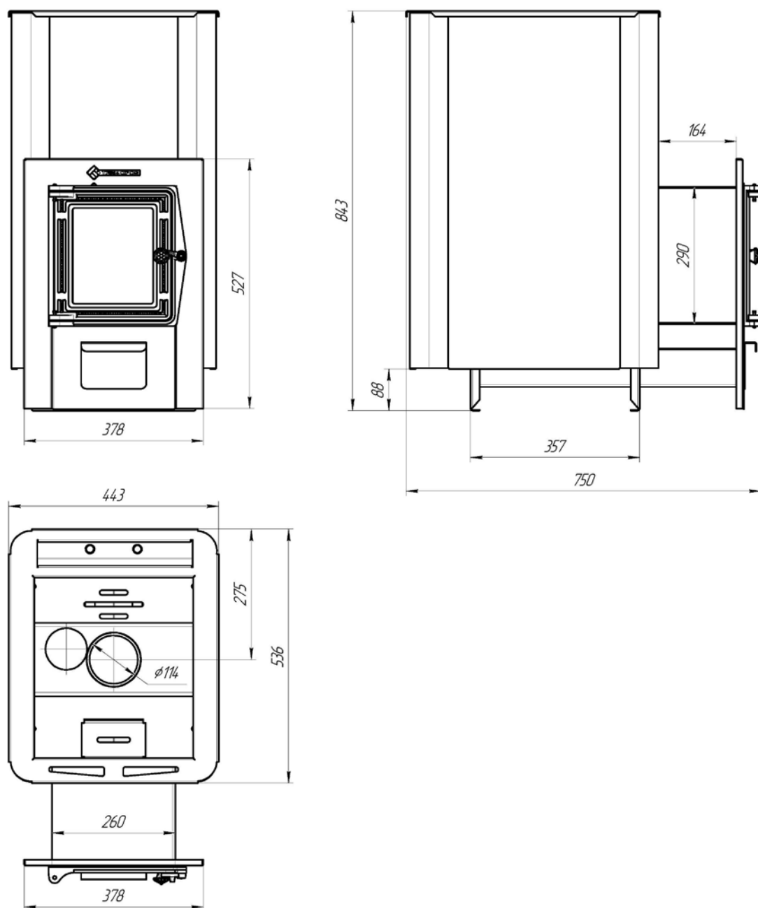
Габаритные размеры печи «ДоброПар 14-18» (чугунная дверца)
