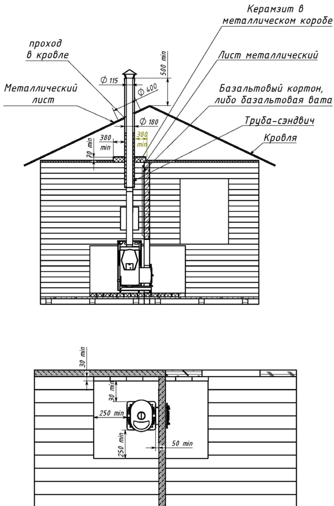
Рисунок 2б – Схема монтажа печи (виды сбоку и сверху)
