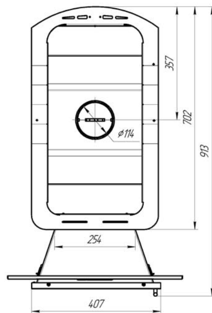
Габаритные размеры печи «Конвектика 26 Плазма»
