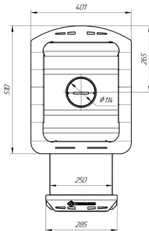
Габаритные размеры печи «Конвектика 12»
