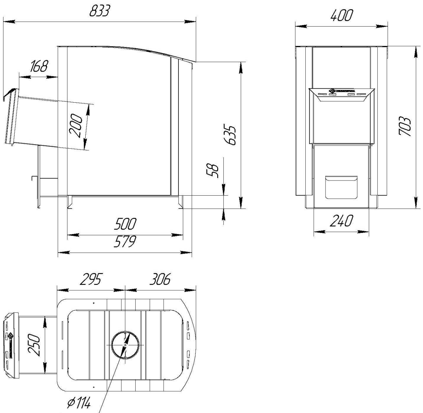
Габаритные размеры печи «Конвектика 16»
