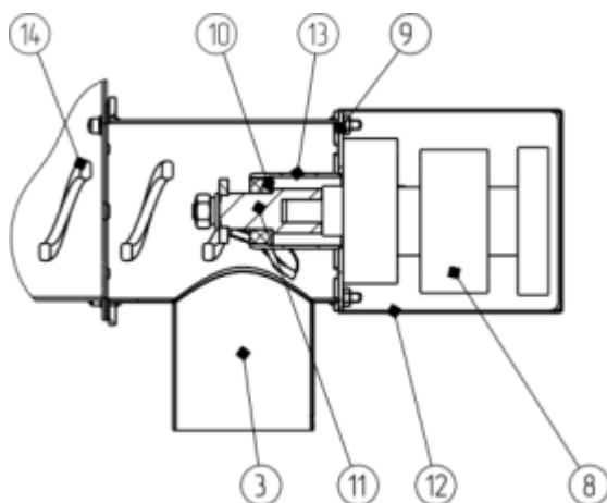
Горелочное устройство (16)
