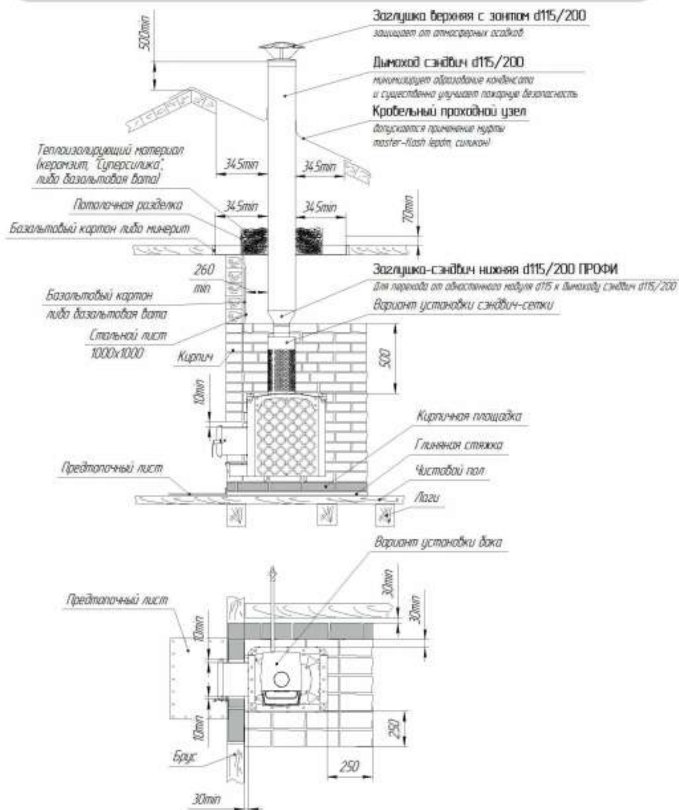
Рисунок 5а - Схема установки печи с кирпичной кладкой
