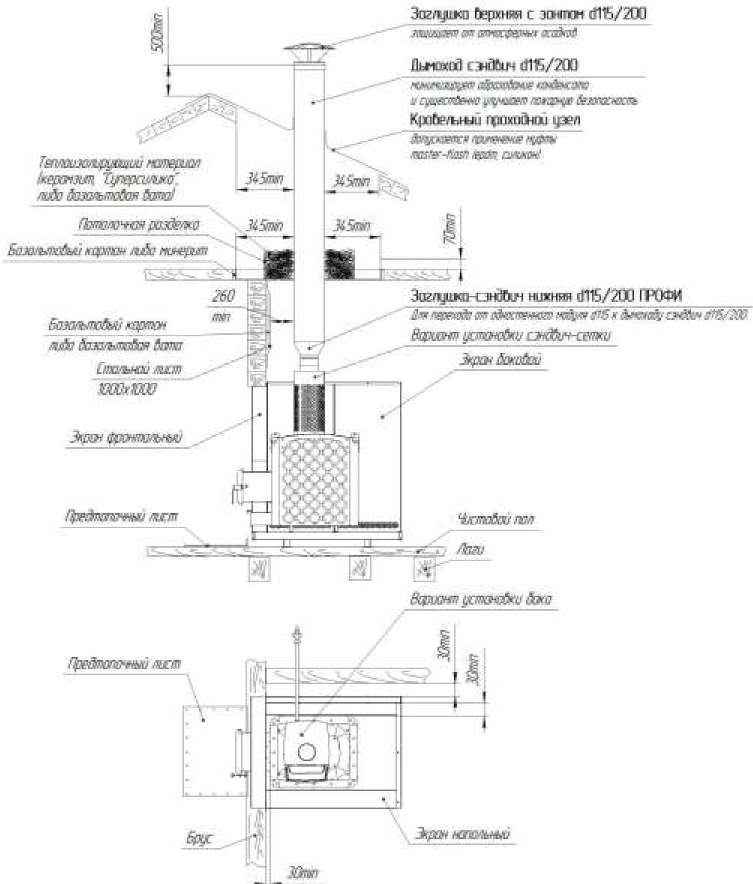
Рисунок 56 - Схема установки печи с защитными экранами
