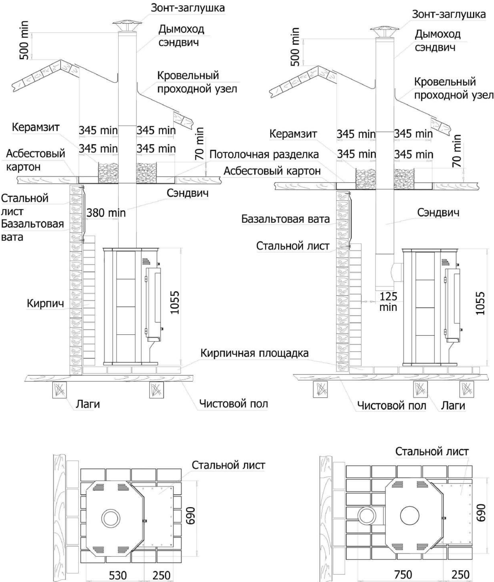
Рис. Схема установки камина и монтаж дымохода
