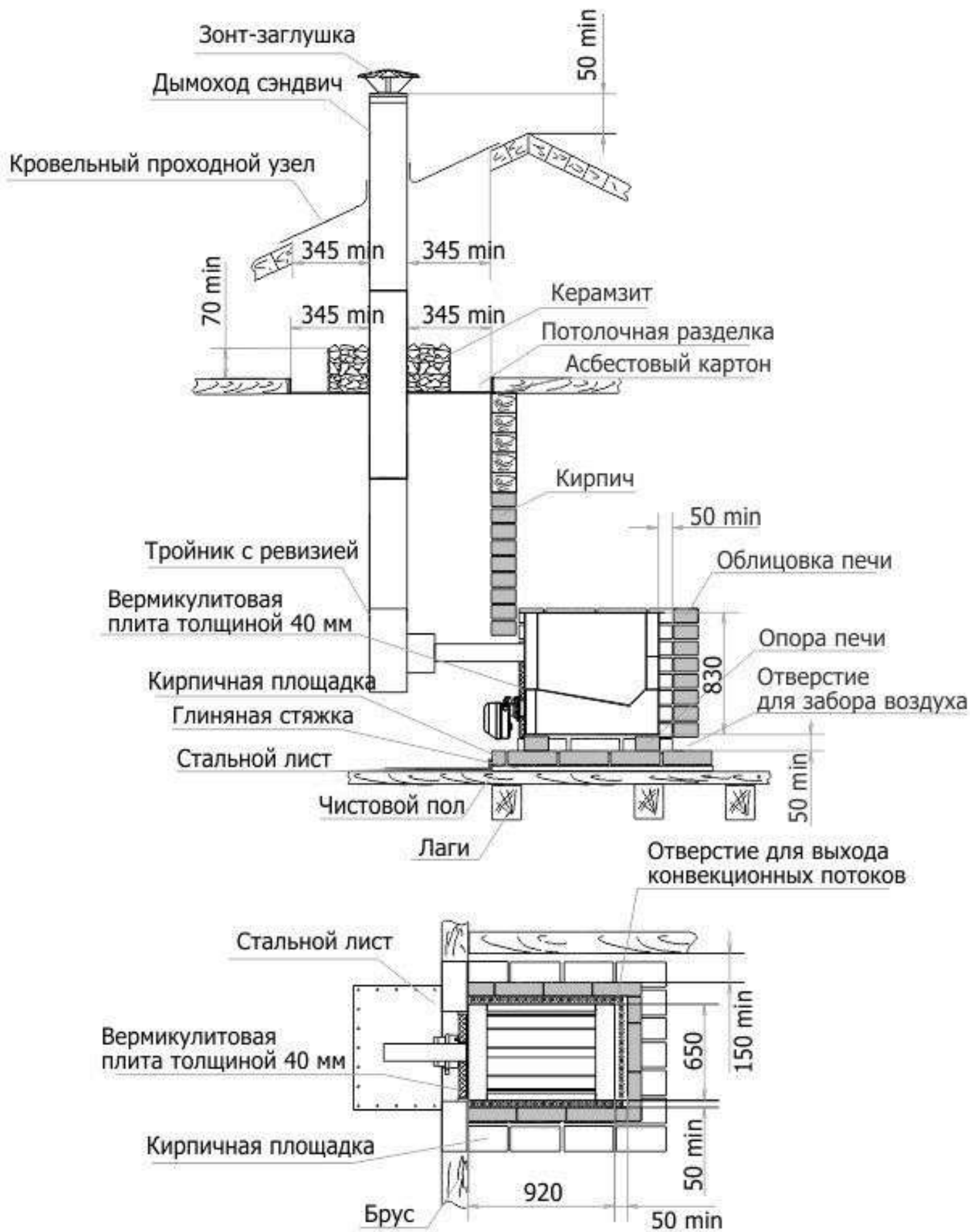
Рекомендуемая схема установки печи «КомПАР»
