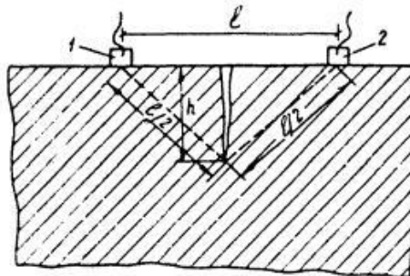
Рисунок 3 – Схема измерения глубины трещины
