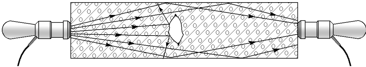
Рисунок 2 – Определение дефекта в бетоне теньевым методом.
