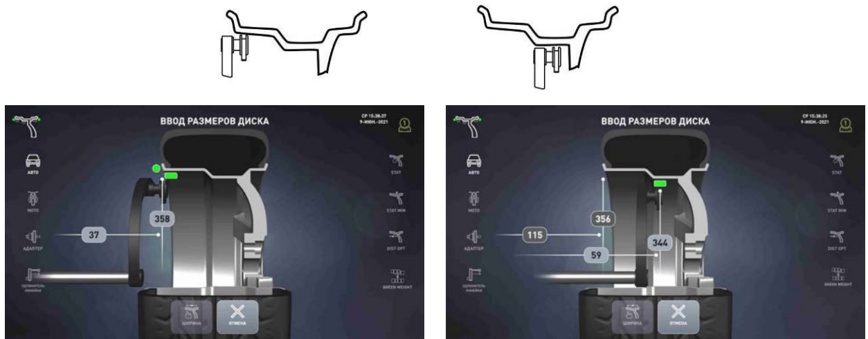
а б Рисунок 6.9 – Ввод размеров
