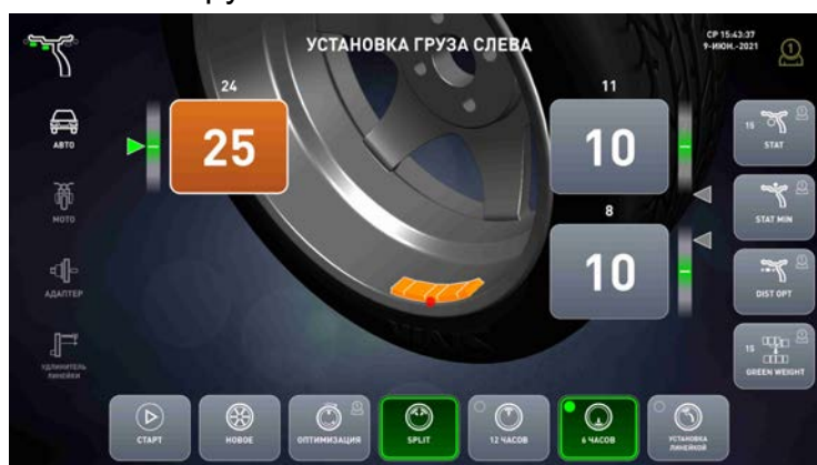
Рисунок 7.5 – Экран установки грузов в режиме Split
